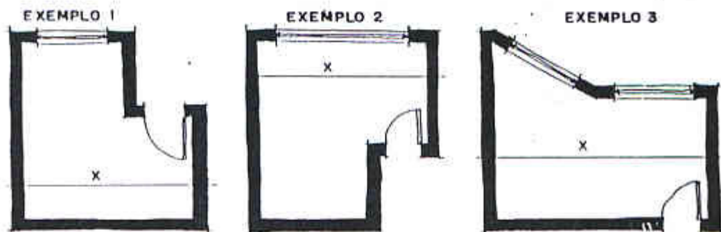
FIG. 9 - EXEMPLOS DE LARGURAS DE COMPARTIMENTOS A SEREM CONSIDERADAS PARA O CÁLCULO DO VÃO DE ILUMINAÇÃO.
