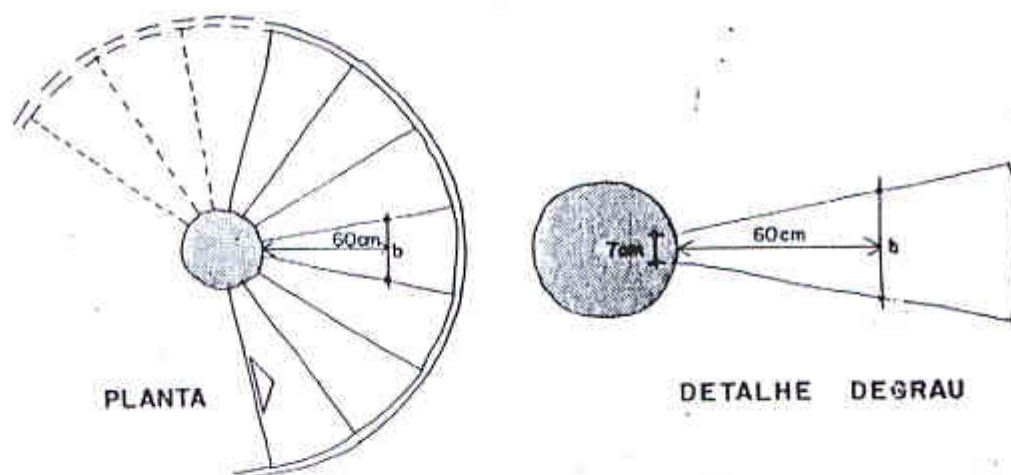
FIG.2- DIMENSIONAMENTO DAS ESCADAS EM LEQUE.
