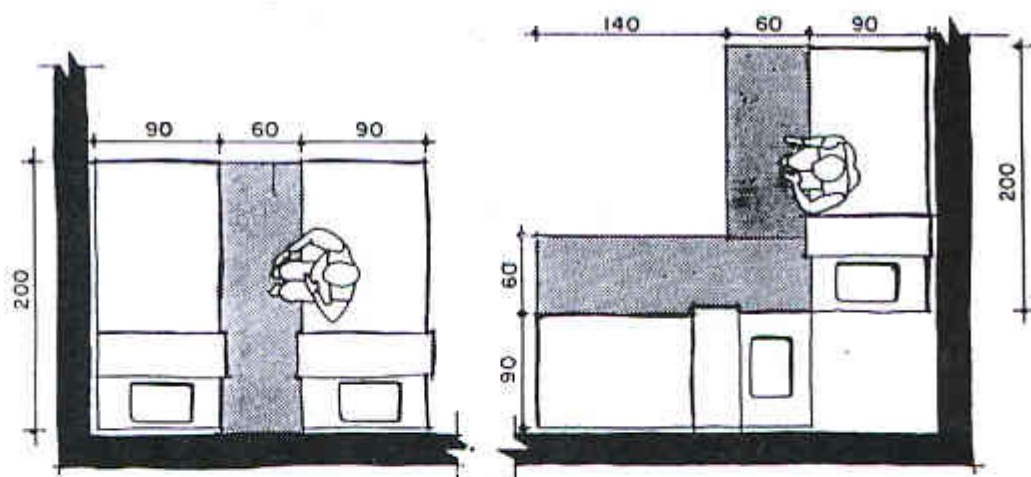
FIG 13 - CAMAS, COM FAIXAS DE ACESSO LIVRE.
