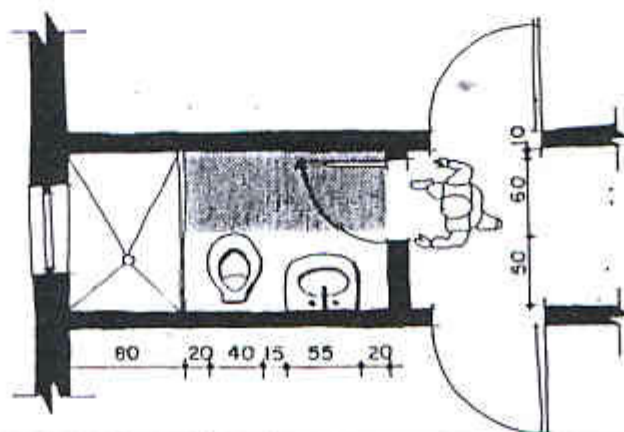
FIG.23 - COMPARTIMENTO SANITÁRIO, COM FAIXA DE ACESSO LIVRE.
