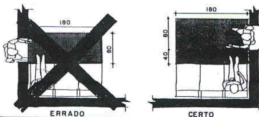
FIG.24- EXEMPLO DE SOFÁ, COM FAIXA DE ACESSO LIVRE COINCIDENTE COM CIRCULAÇÃO DE PORTA.
