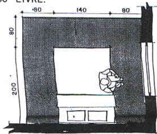
FIG.21 - CAMA DE APARTAMENTO CONJUGADO, COM FAIXA DE ACESSO LIVRE.
