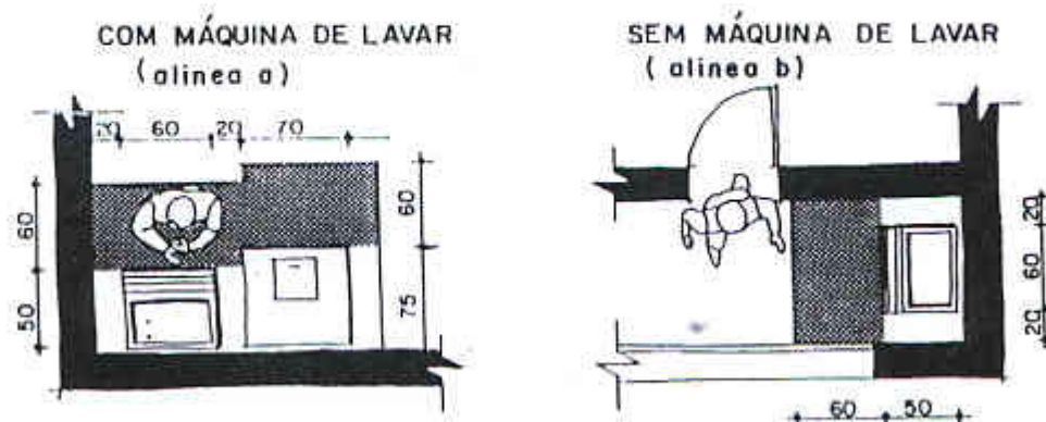
FIG.17- ÁREAS DE SERVIÇO, COM FAIXA DE ACESSO LIVRE.
