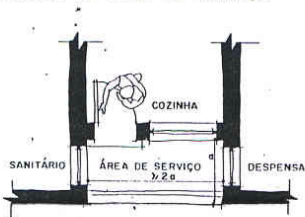
FIG.8- VENTILAÇÃO E ILUMINAÇÃO DE COMPARTIMENTO ATRAVÉS DE ÁREA DE SERVIÇO.
