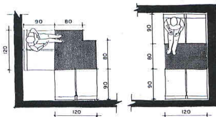
FIG. 11 - SOFÁS COM ACESSO LIVRE.
