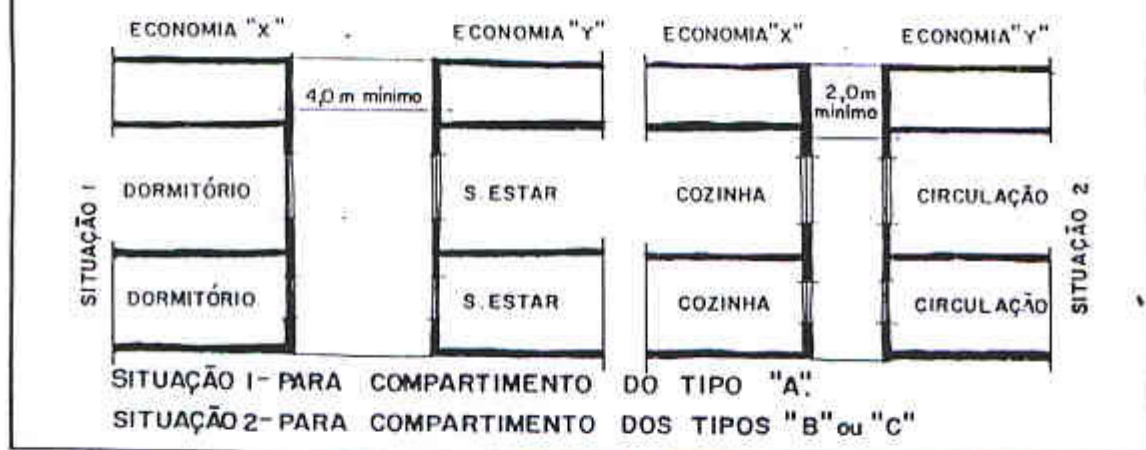
FIG.6- DISTÂNCIAS MÍNIMAS ENTRE ABERTURAS DE ECONOMIAS DISTINTAS.
