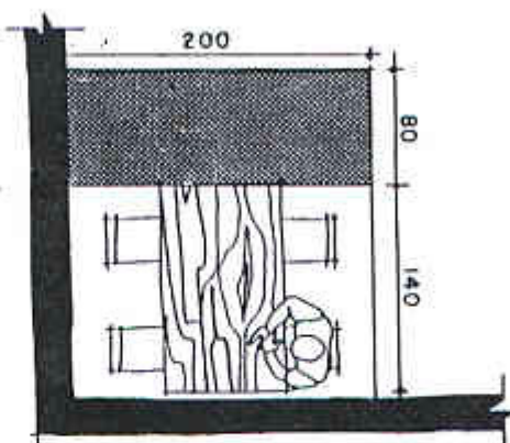
FIG.12- CONJUNTO DE MESA E QUATRO CADEIRAS, COM FAIXA DE ACESSO LIVRE.
