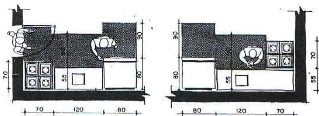
FIG. 16- EQUIPAMENTO DE COZINHA, COM FAIXA DE ACESSO LIVRE.
