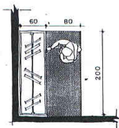
FIG.22- ROUPEIRO DE APARTAMENTO CONJUGADO, COM FAIXA DE ACESSO LIVRE.
