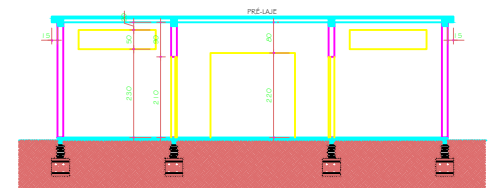
CORTE A-A' Escala: 1:50
