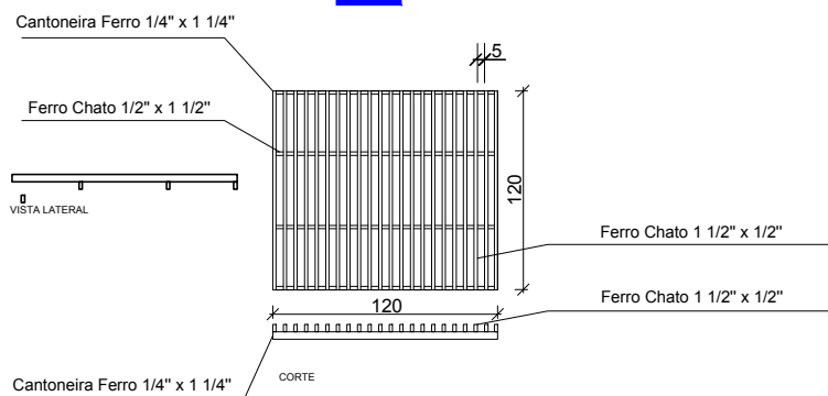
DETALHE FERRAGEM - TAMPA SEM ESCALA
