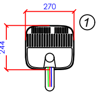
Vista Superior
