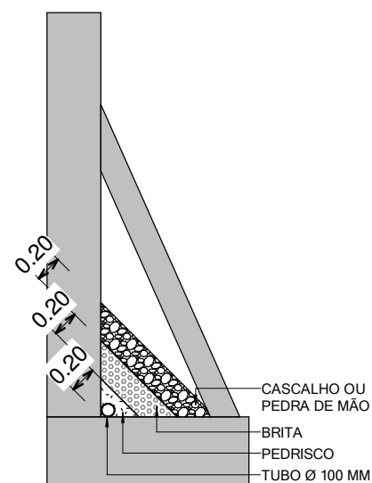
04 DET - DRENO 1 : 50
