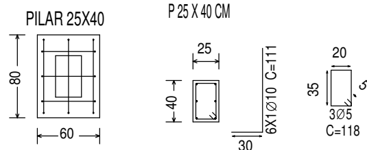
06 SAPATAS 1 : 50
