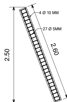
05 PILAR INCLINADO 1 : 50
