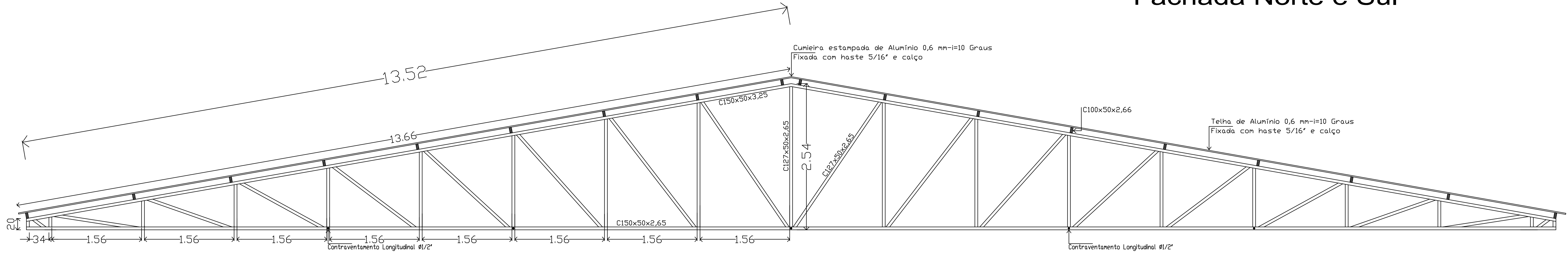
Detalhe da Tesoura Metálica
