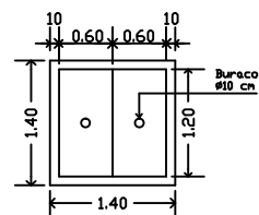
Boca-de-Lobo Planta Baixa Tampas Escala 1 : 50 Altura=7cm
