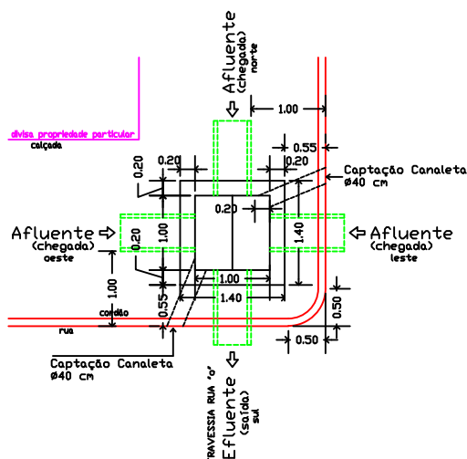
Boca-de-Lobo - A1 Planta Baixa em Esquina Escala 1 : 50
