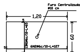
Boca-de-Lobo Ferragem-Tampa Escala 1 : 25 Altura= 7 cm
