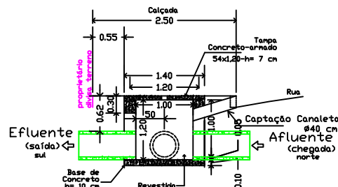
Boca-de-Lobo Corte em Esquina Escala 1 : 50
