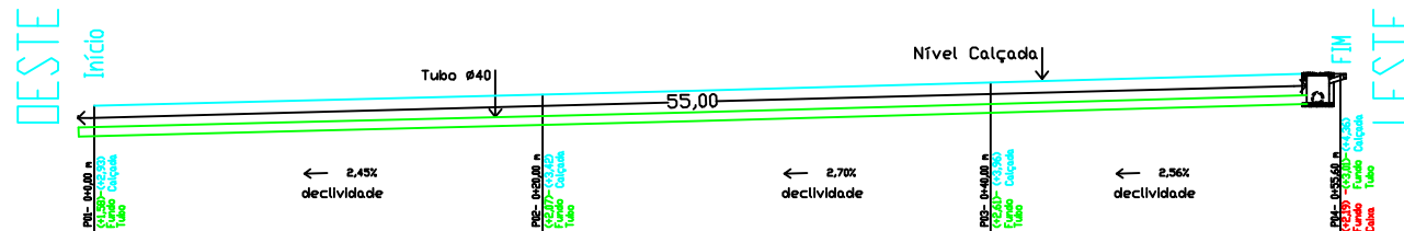
CORTE LONGITUDINAL DO ESGOTO PLUVIAL DA RUA " S " CALÇADA DIREITA - SUL ESCALA 1 : 250
