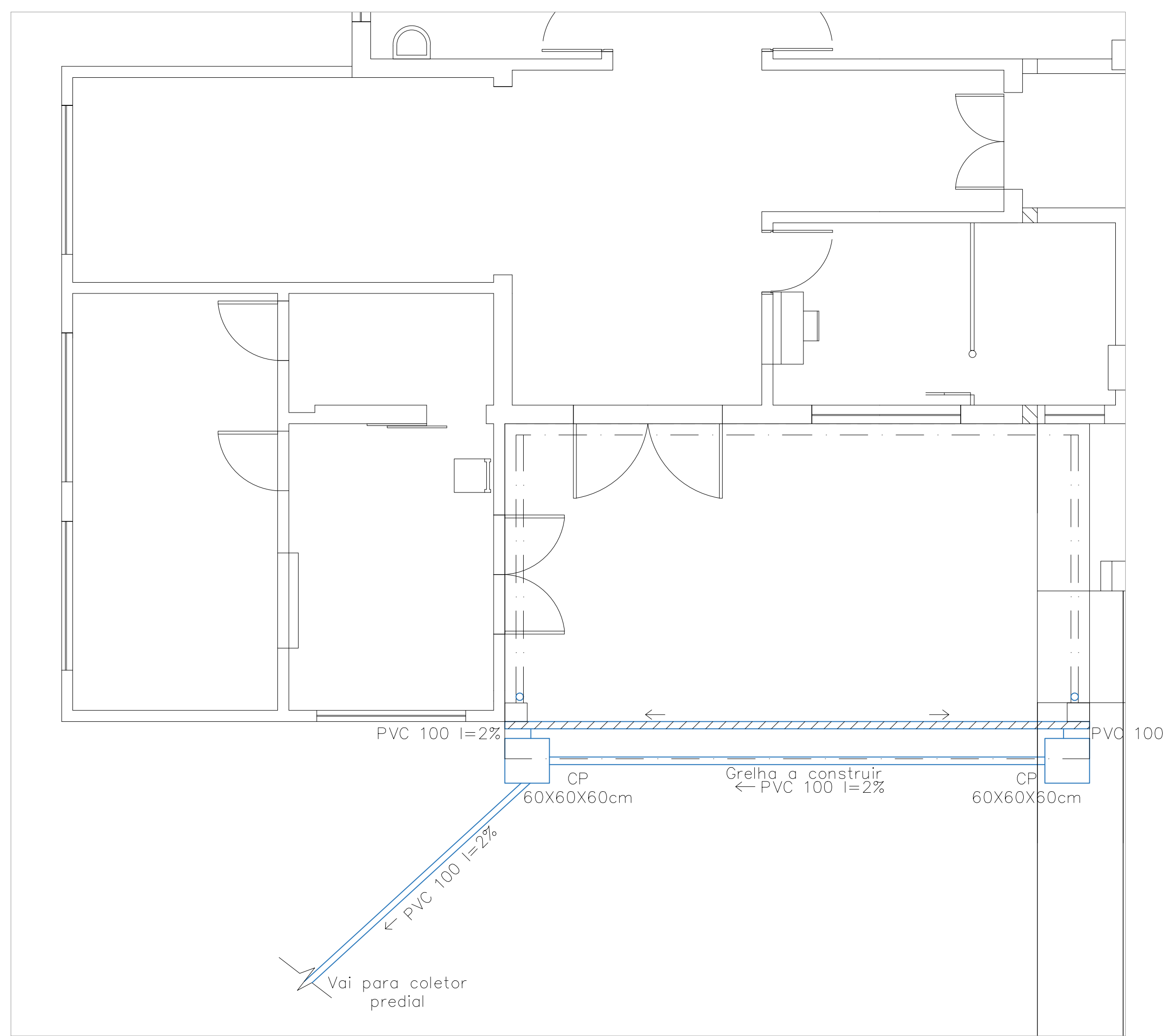
11 PROJETO PLUVIAL
