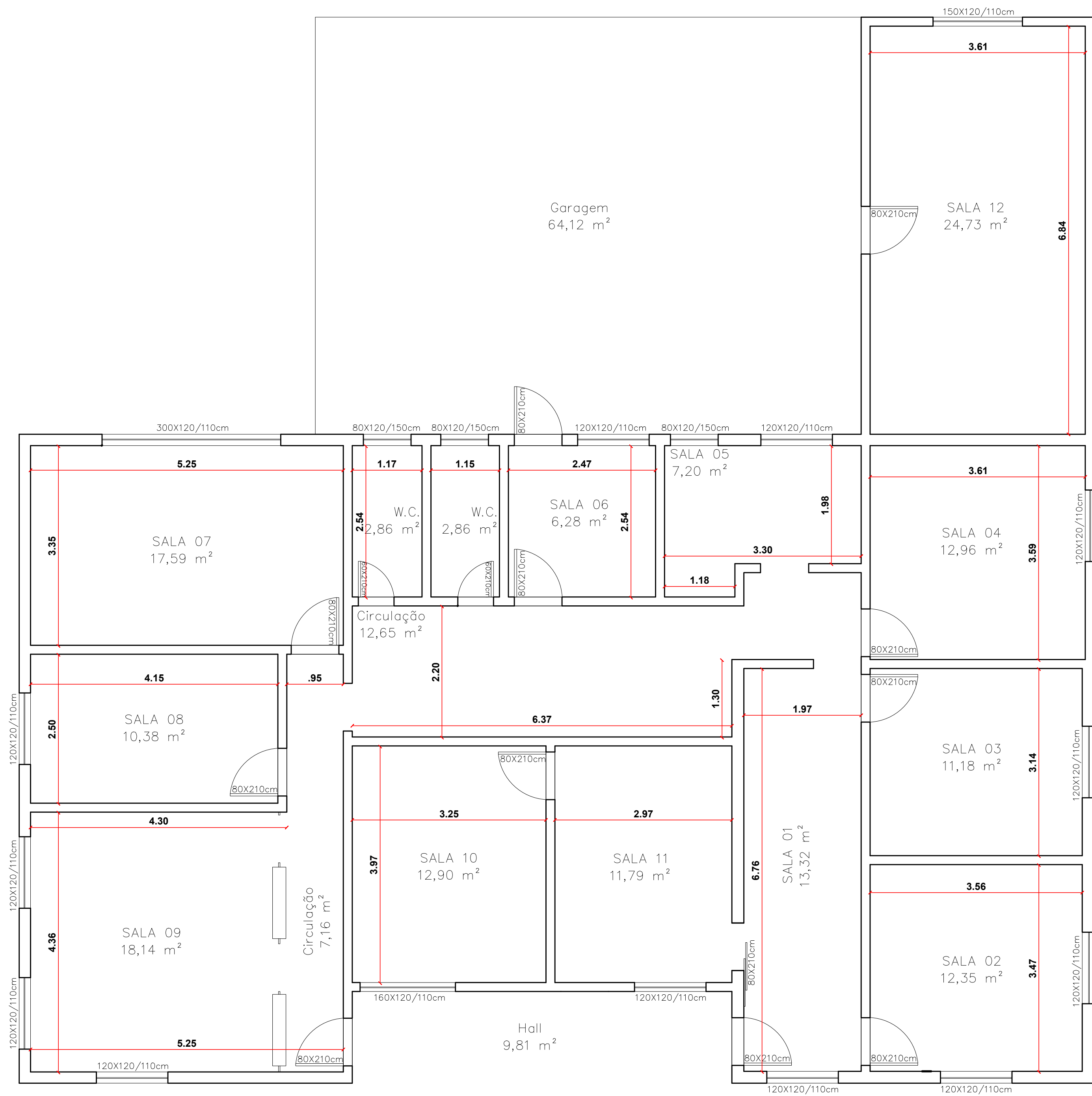
01 PLANTA BAIXA EXISTENTE ESC.: 1:50
