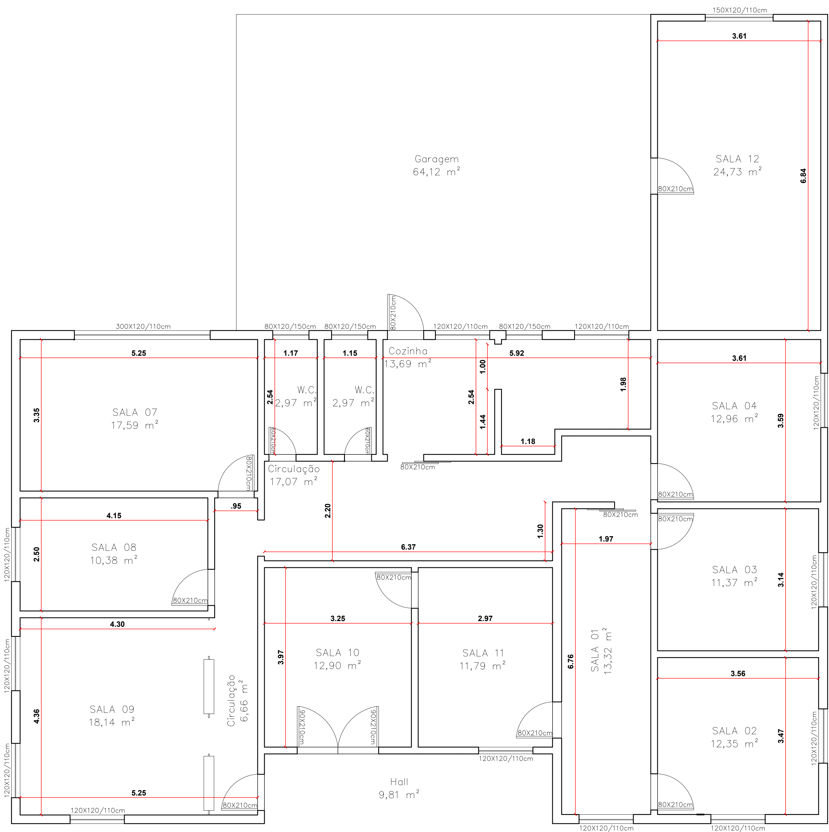
02 PLANTA BAIXA PRETENDIDA ESC.: 1:50
