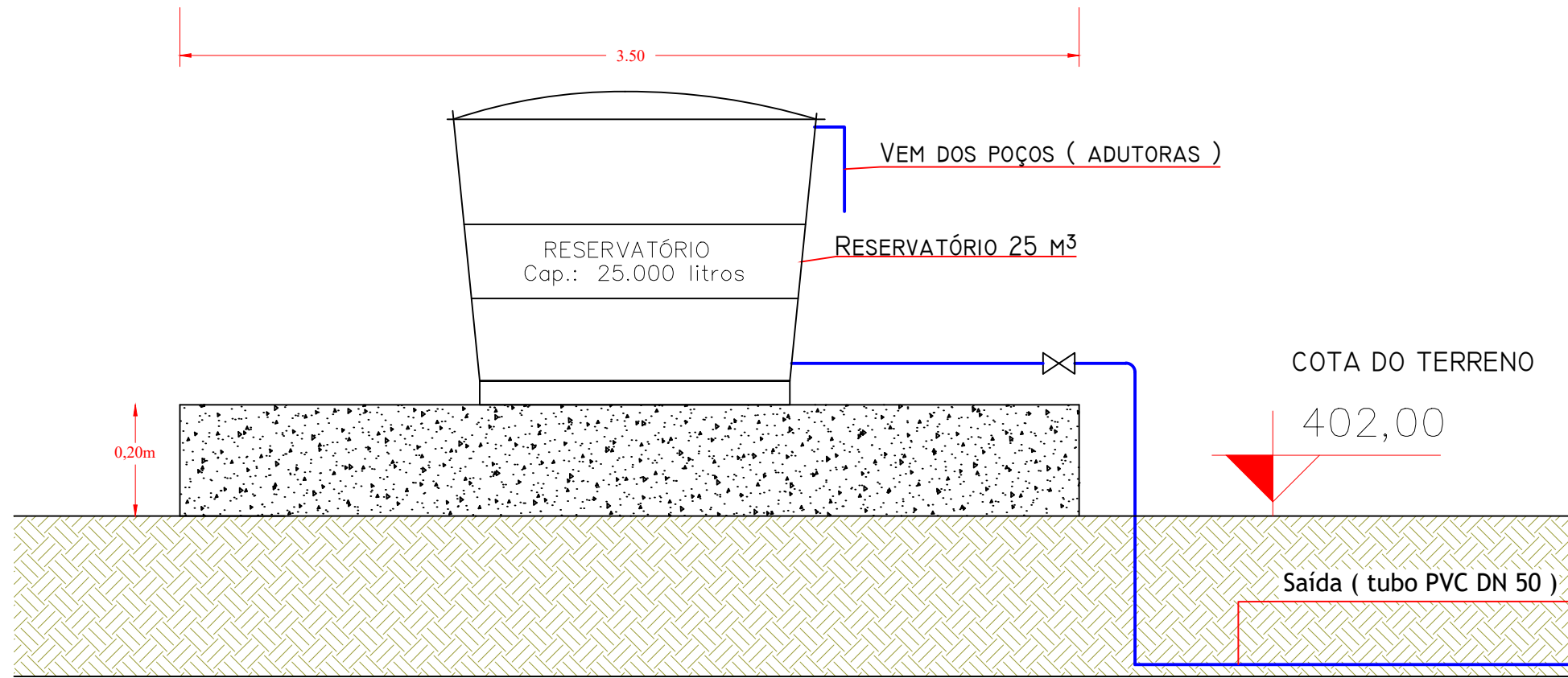
INSTALAÇÃO DO RESERVATÓRIO
