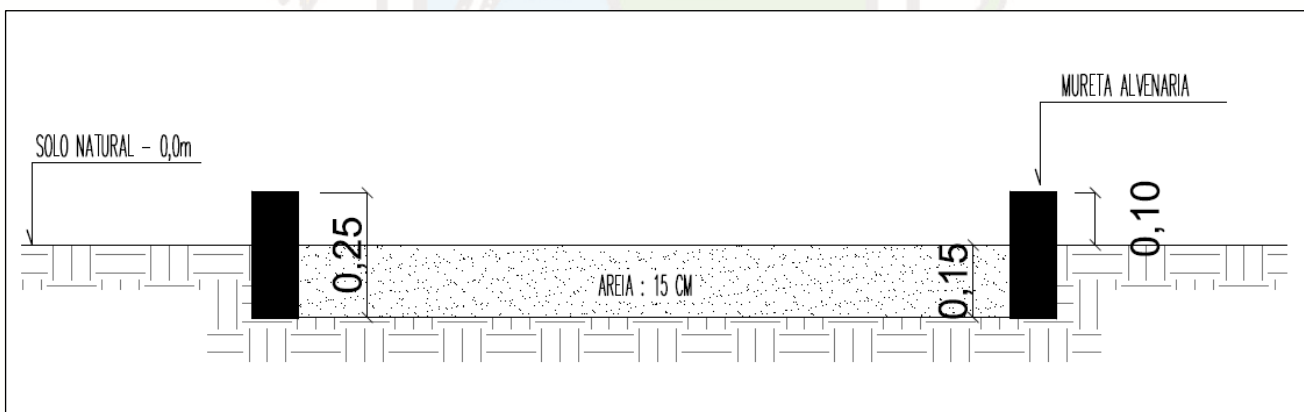
Figura 01: Croqui de execução da caixa de areia.
