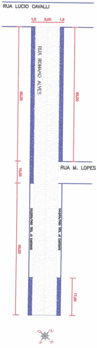
PLANTA BAIXA DA RUA ETC - TOTAL 180,00m AREA 1.170,00m²
