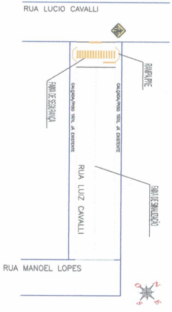
PLANTA BAIXA DA RUA 01 ESCALA 1:400
