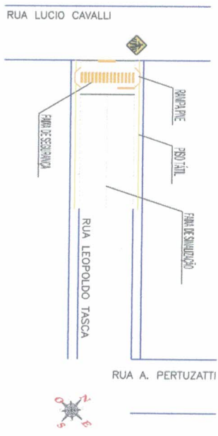
PLANTA BAIXA DA RUA 01 ESCALA 1:400
