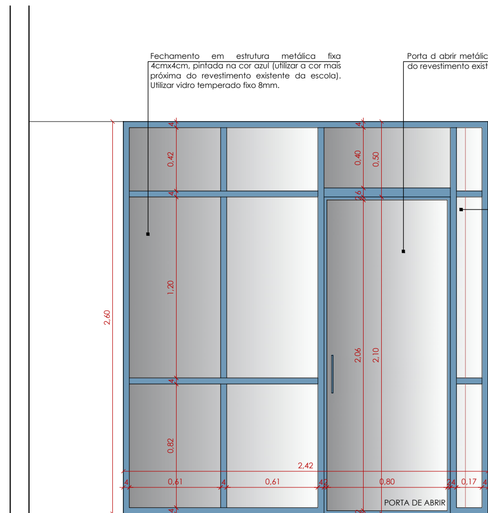
VISTA B - frontal Esc.: 1/25
