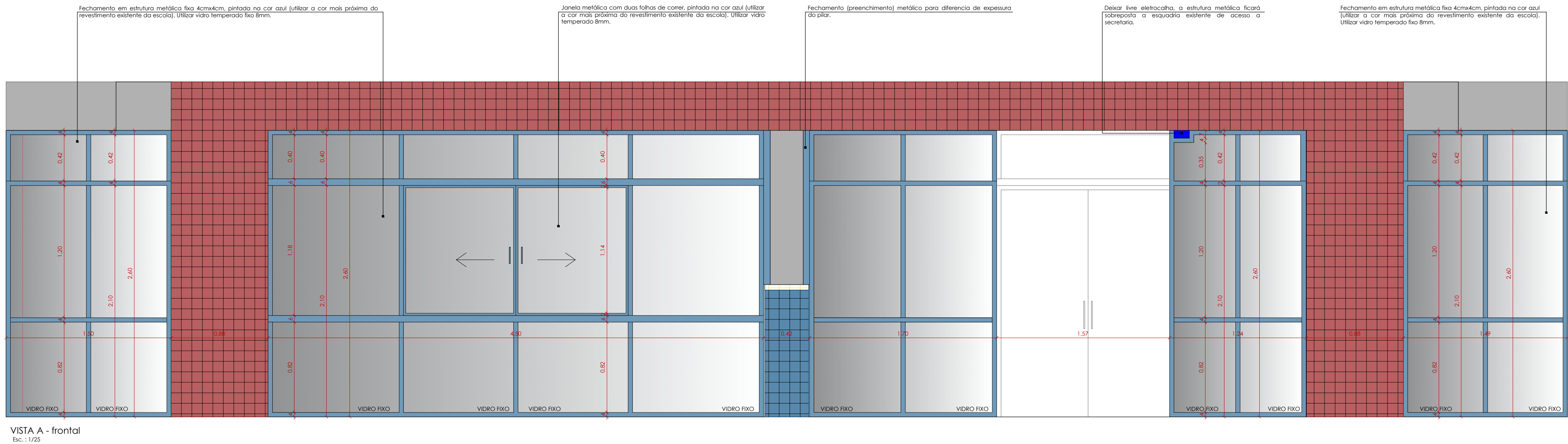
VISTA A - frontal Esc.: 1/25
