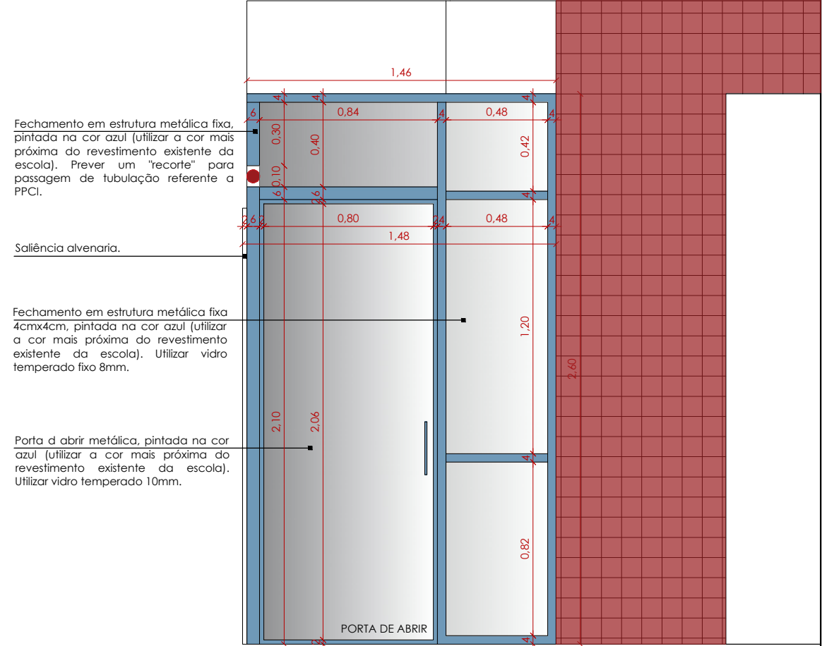
VISTA D - frontal Esc.: 1/25
