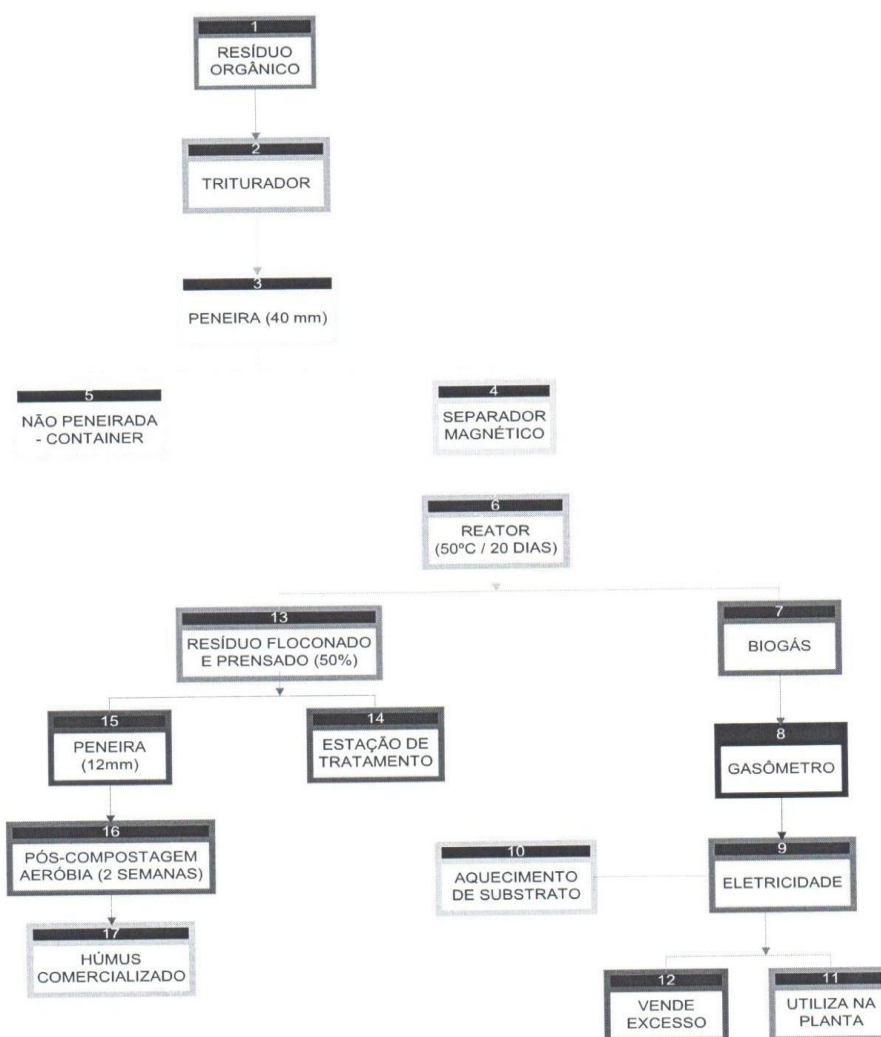
Figura 23 Fluxograma do processo contemplado na tecnologia Dranco
