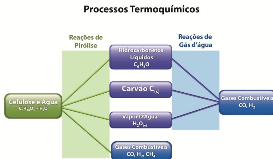
Figura 19: Sistema Innova – Esquema dos processos termoquímicos
