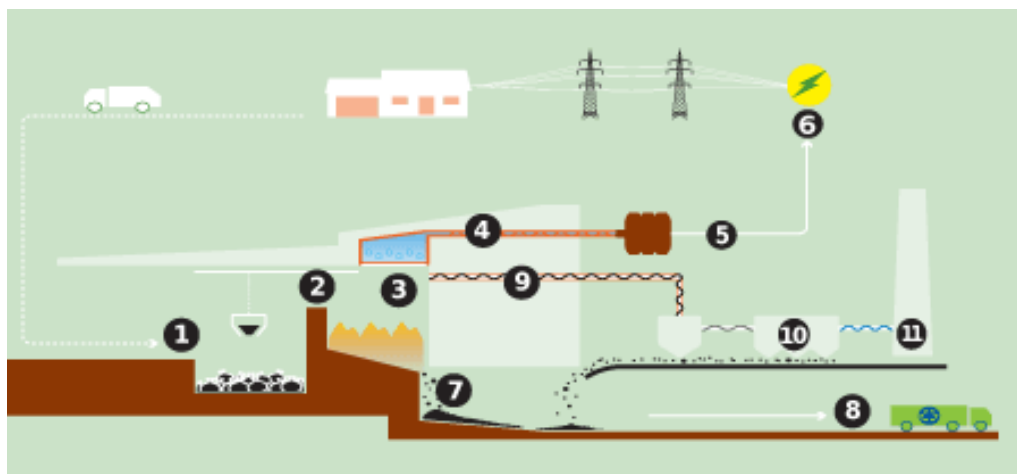
Figura 21: Sistema Covanta – Esquema do processo
