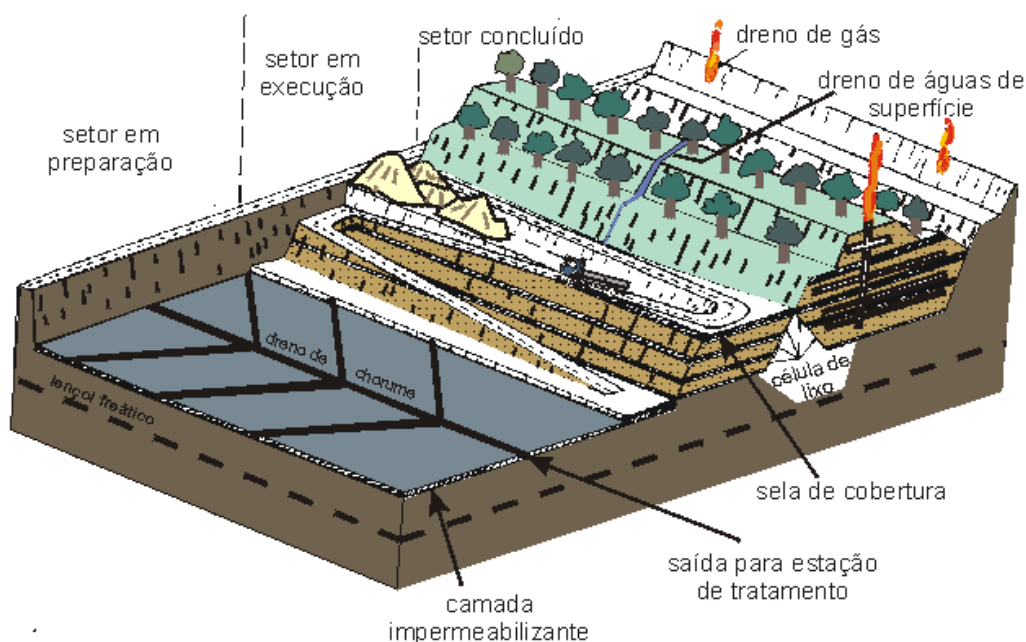
Figura 4: Estrutura padrão de aterros sanitários
