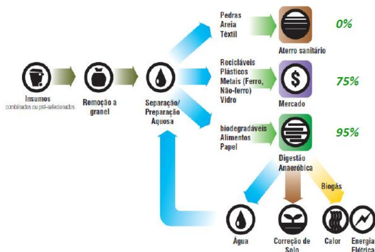
Figura 20: Sistema ArrowBio – Esquema do processo
