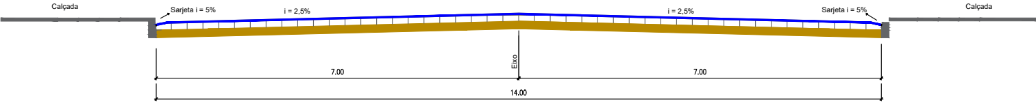
Seção transversal tipo ruas de 14m de largura
