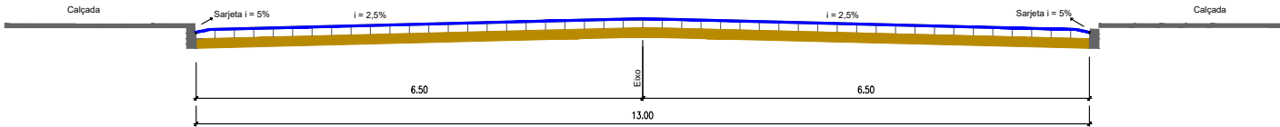
Seção transversal tipo ruas de 13m de largura
