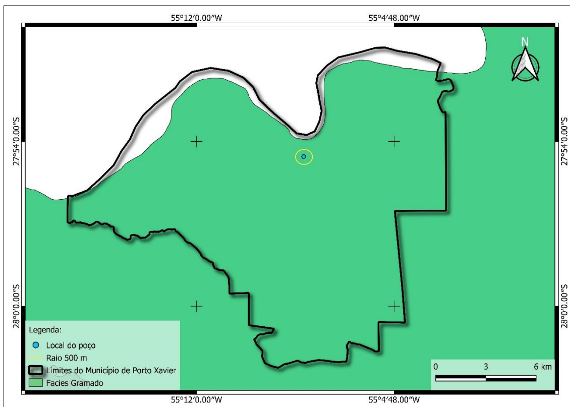
Figura 02. Mapa Geológico do Município de Porto Xavier.
