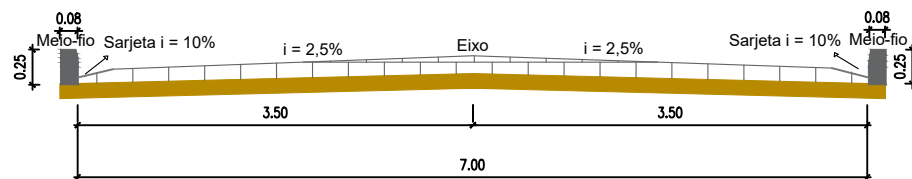
Seção transversal tipo ruas de 7,00m
