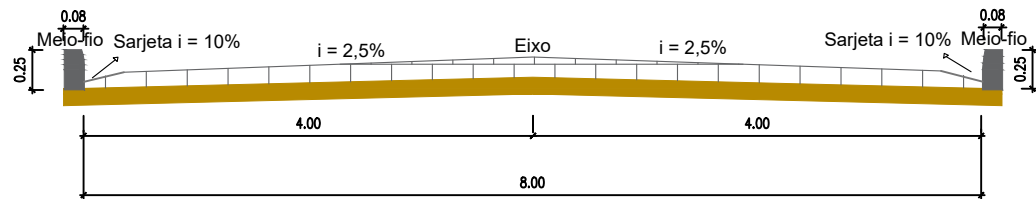
Seção transversal tipo ruas de 8,00m
