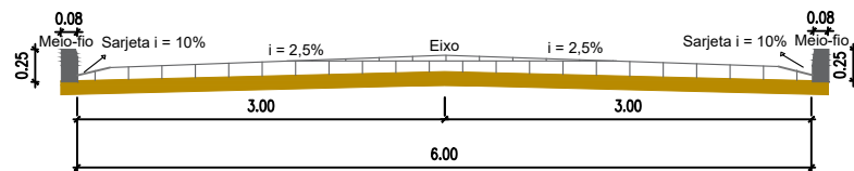
Seção transversal tipo ruas de 6,00m
