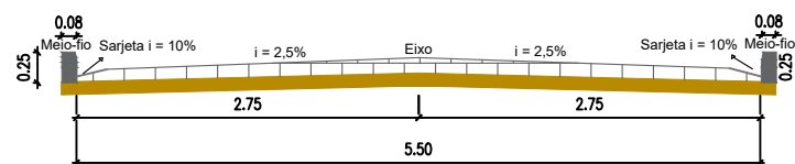
Seção transversal tipo ruas de 5,50m
