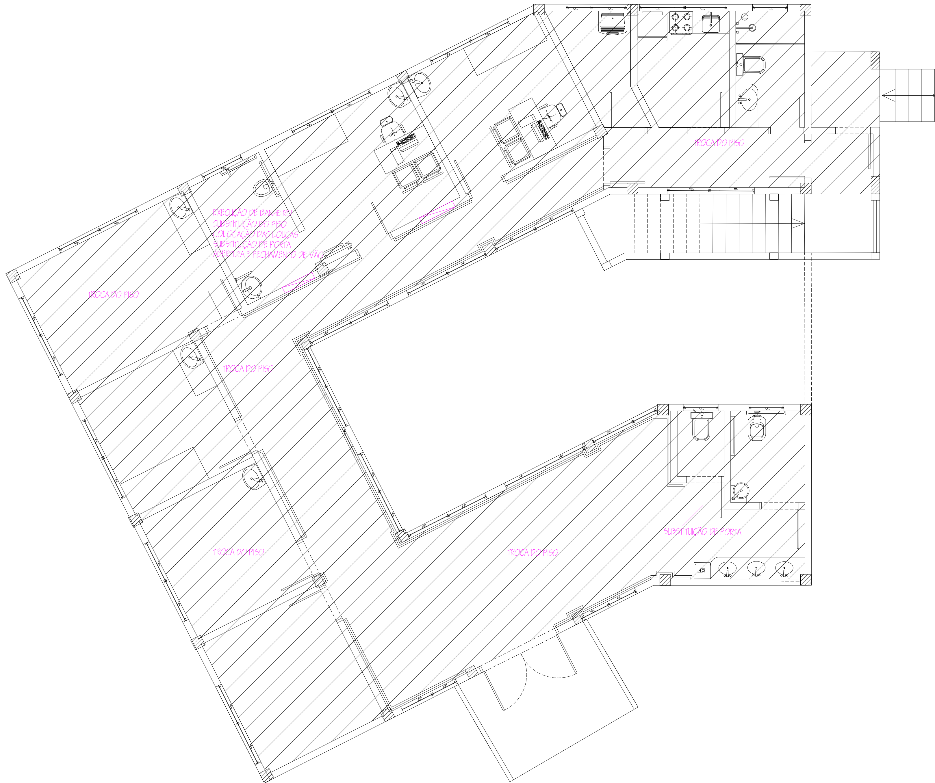
1 REFORMAS PAVIMENTO TÉRREO ESCALA 1:50
