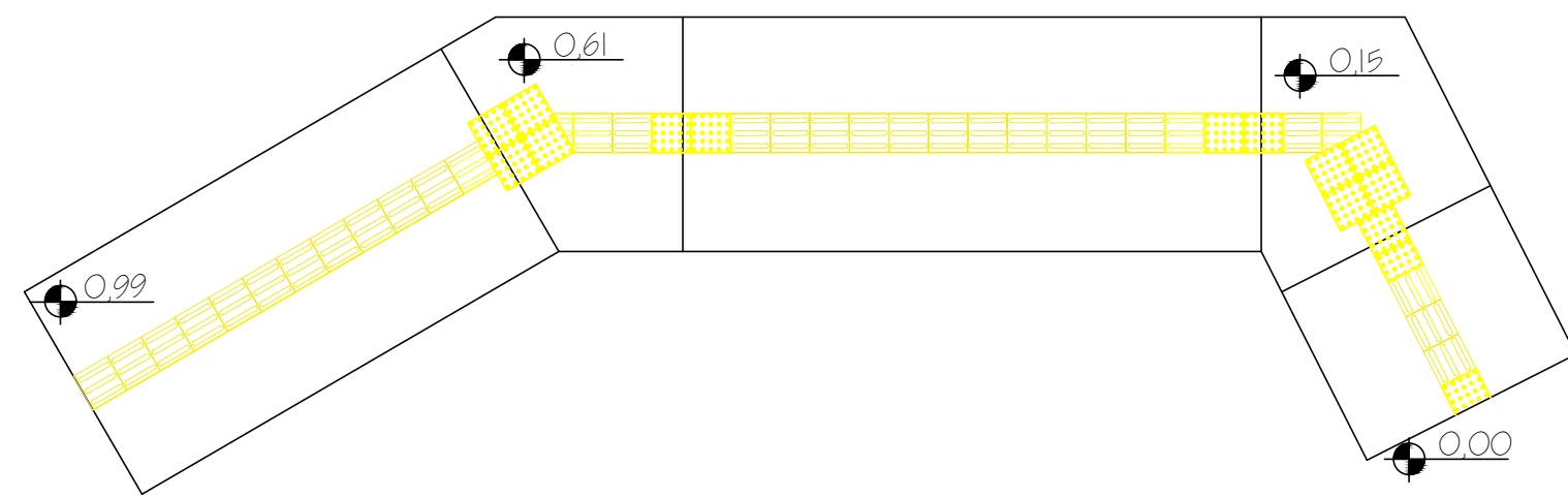
1 DETALHE 01 ESCALA 1:50
