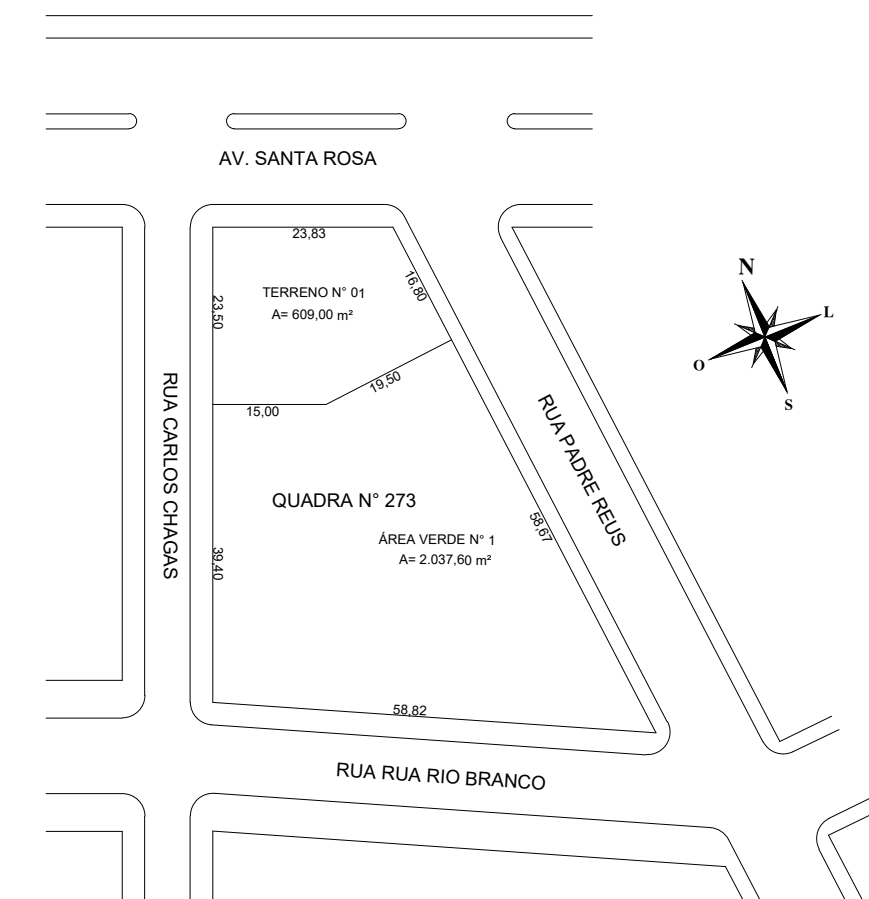
3 PLANTA DE SITUAÇÃO ESCALA 1:1000
