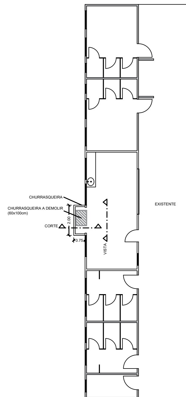
PLANTA BAIXA 1:150
