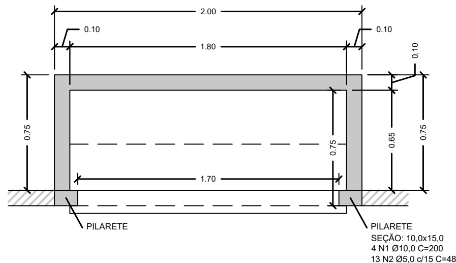
VISTA FRONTAL 1:25
