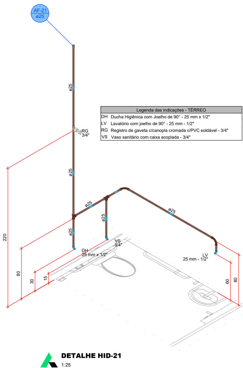
DETALHE HID-21 1:25
