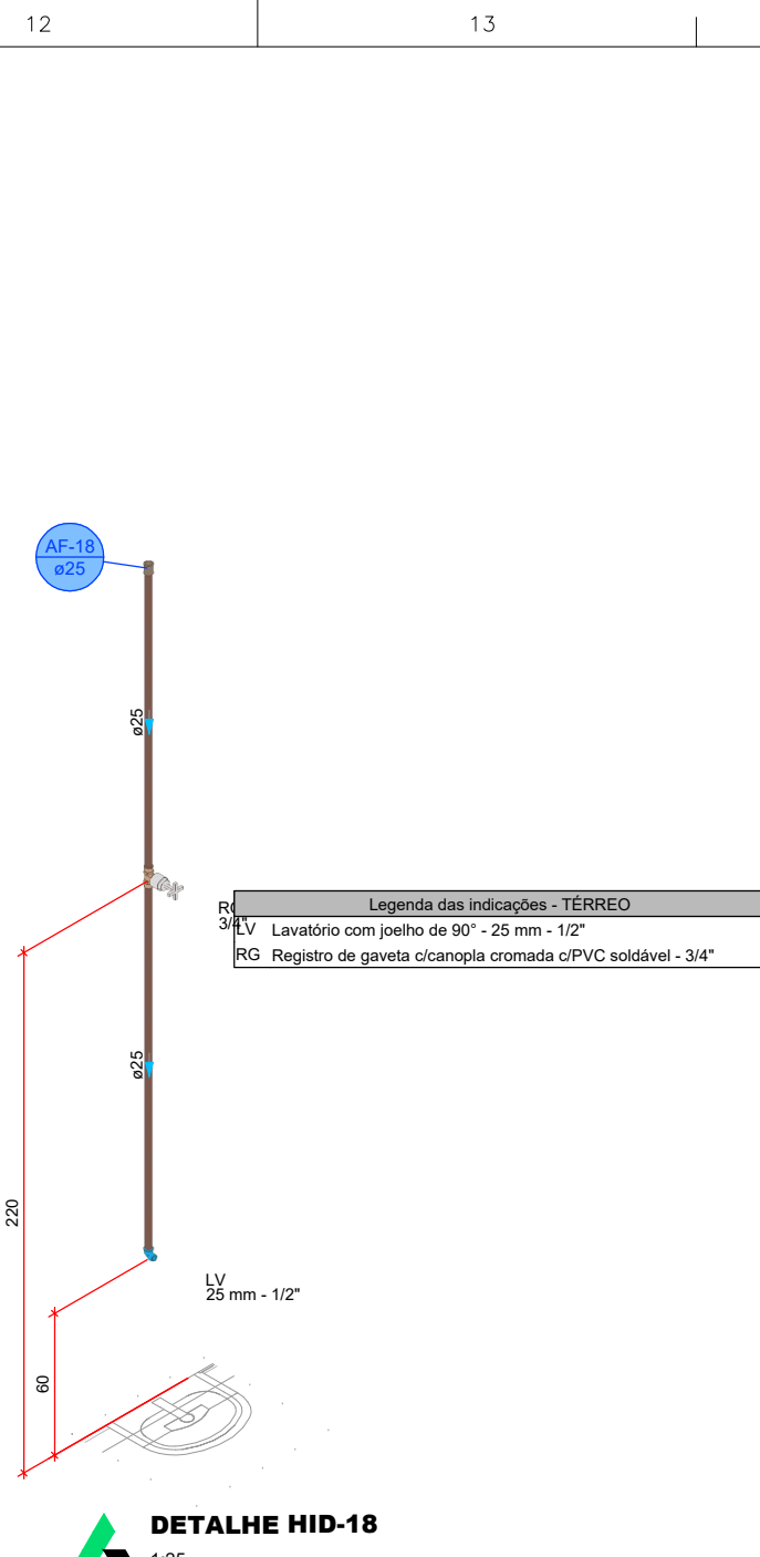
DETALHE HID-18 1:25
