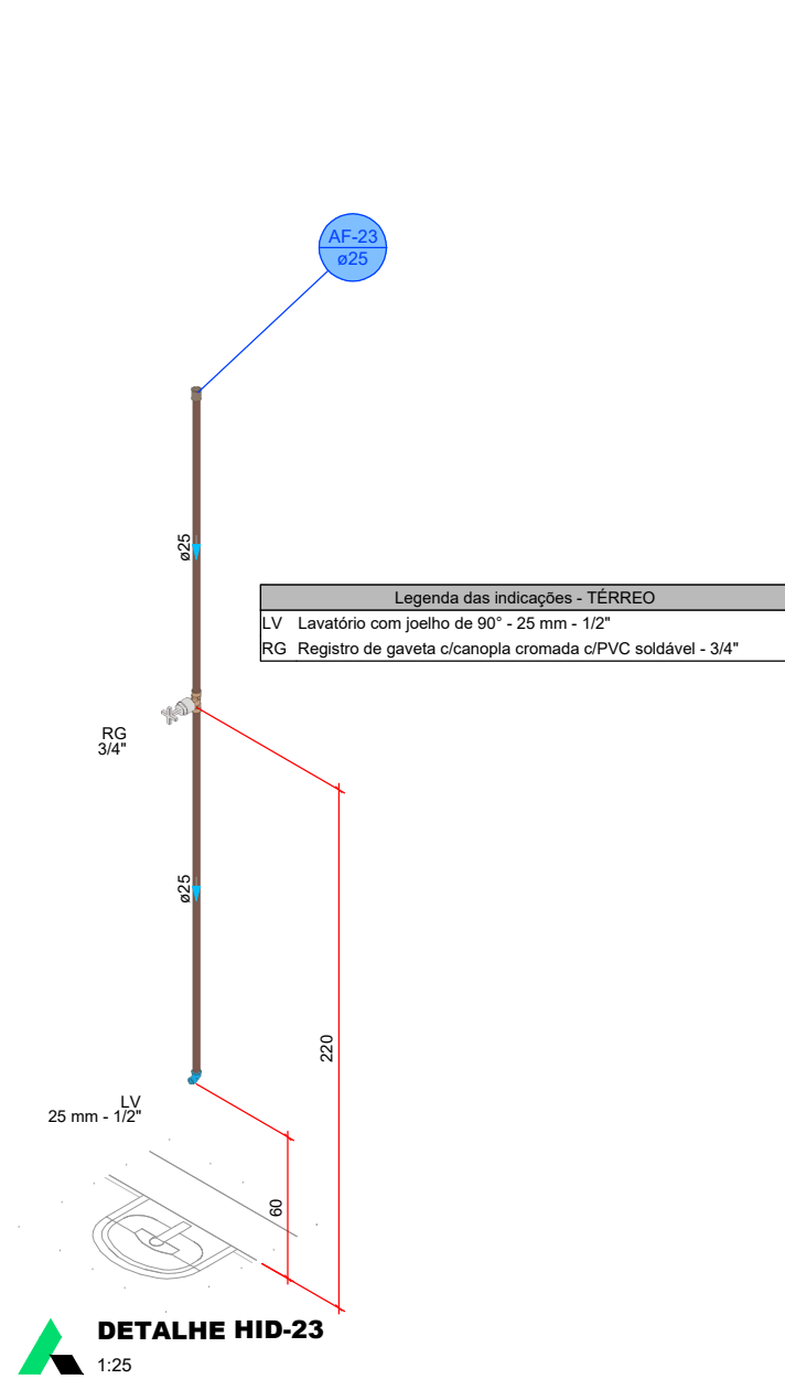
DETALHE HID-23 1:25
