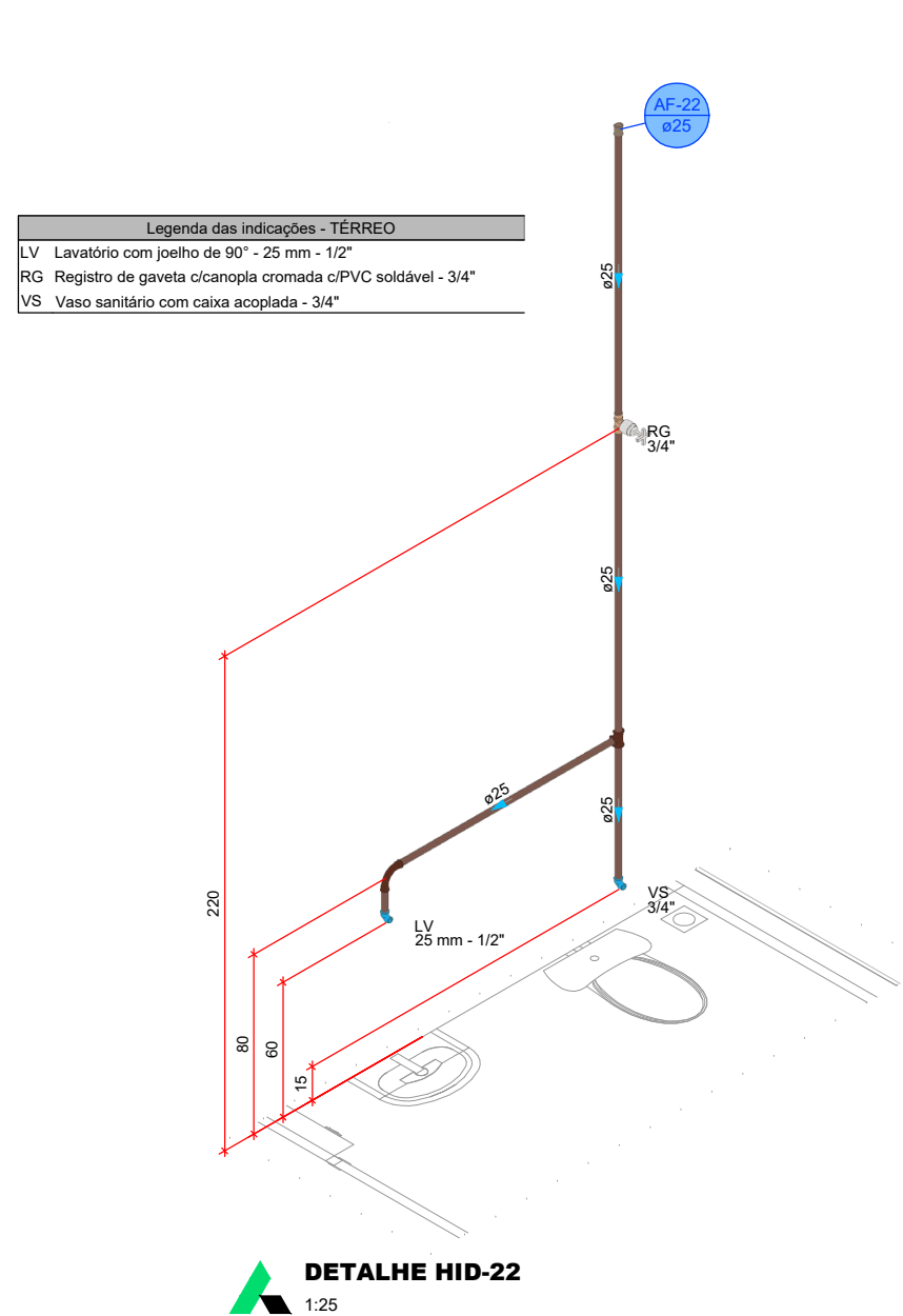
DETALHE HID-22 1:25
