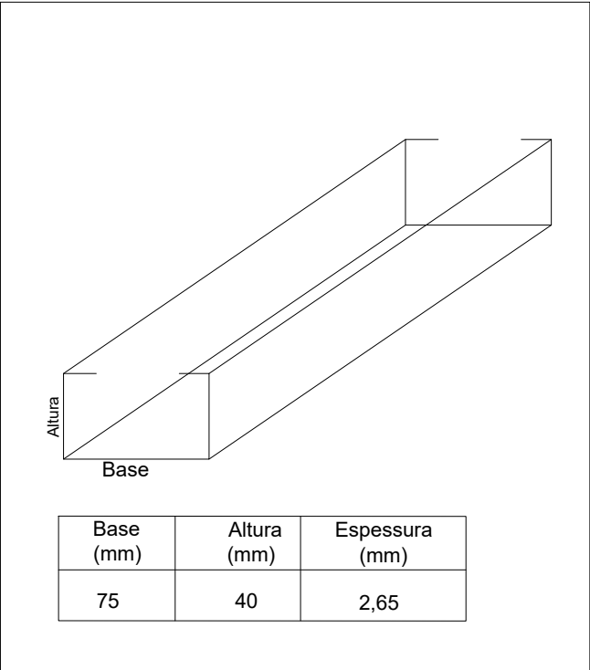
Detalhamento da estrutura metálica
