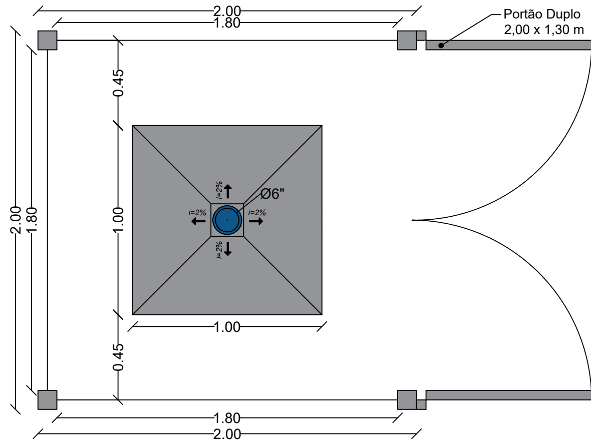
3 Detalhamento Esc.: 1/50
