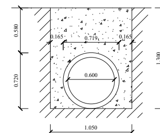
Corte
