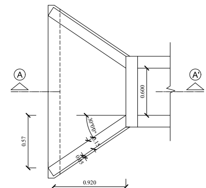
Corte AA'
