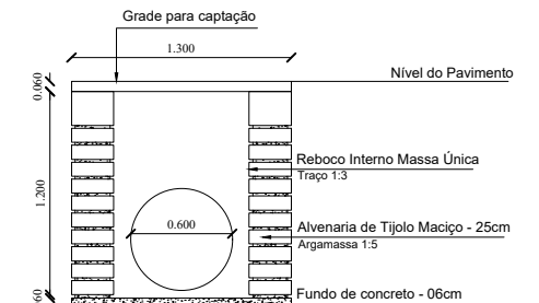
Corte
