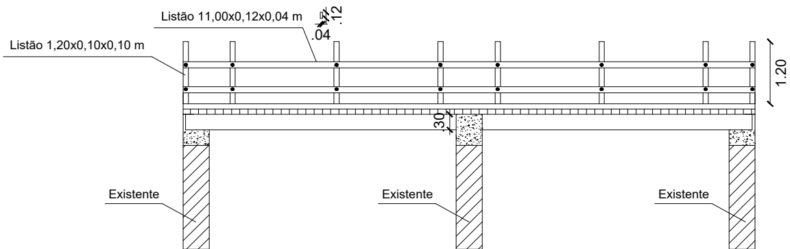
Corte AA
