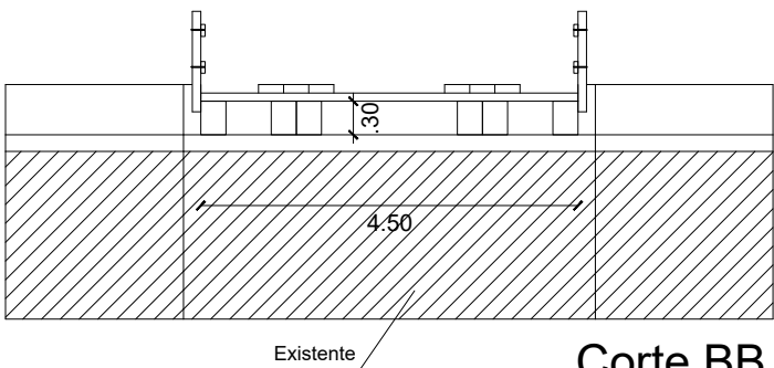
Corte BB
