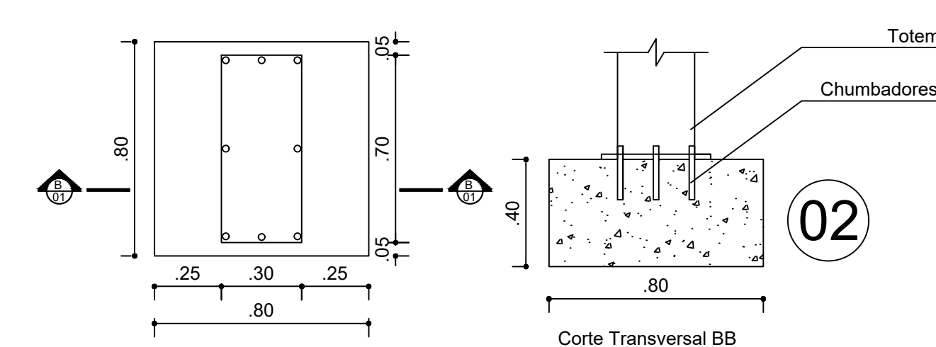
Detalhamento Fundação Totem Escala: 1:20
