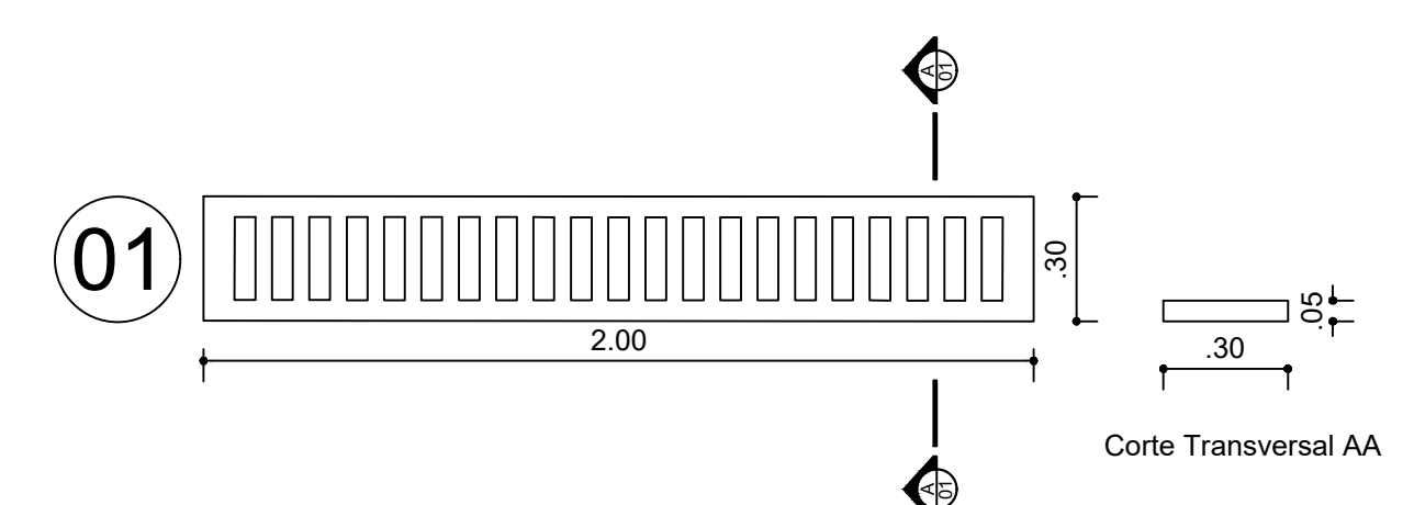
Detalhamento Grade Escala: 1:20
