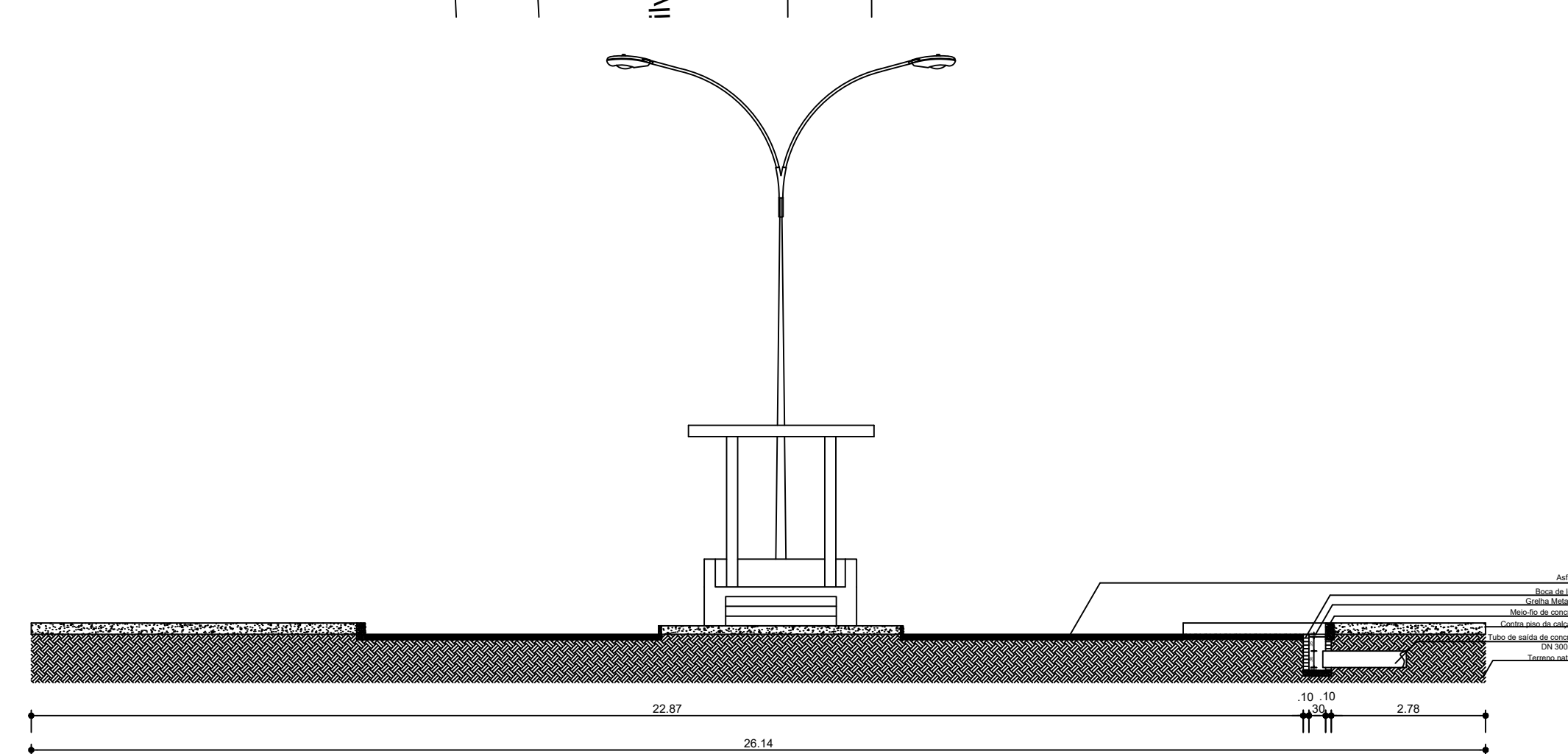
Corte Transversal BB
