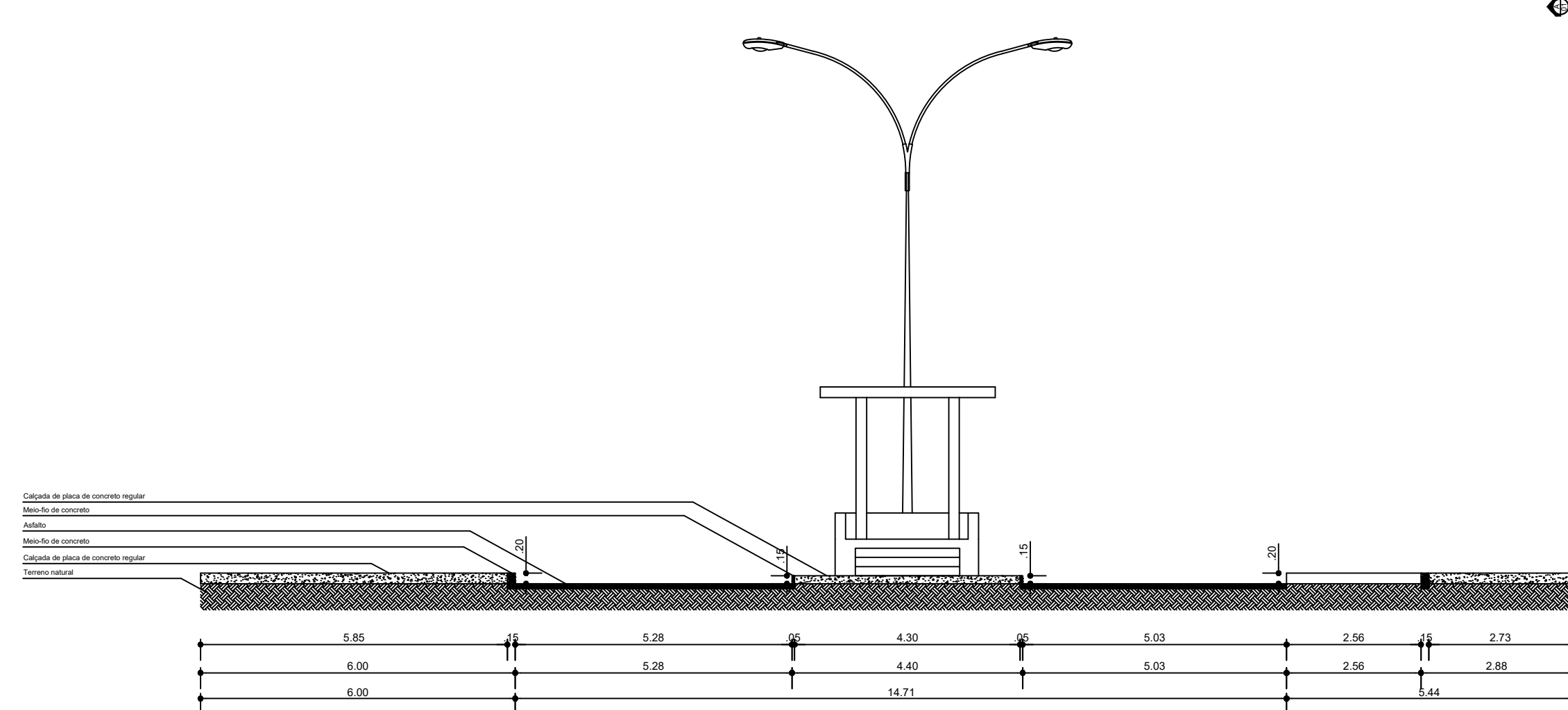
Corte Transversal AA Escala: 1:100
