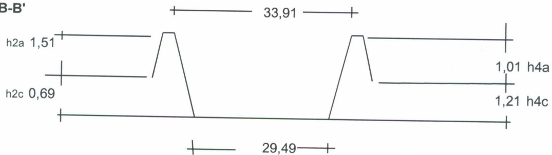
Corte B-B'
