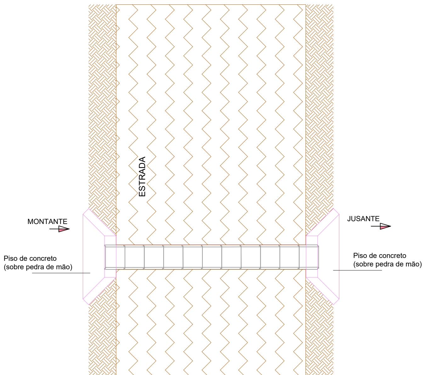
Planta de situação esc 1:150
