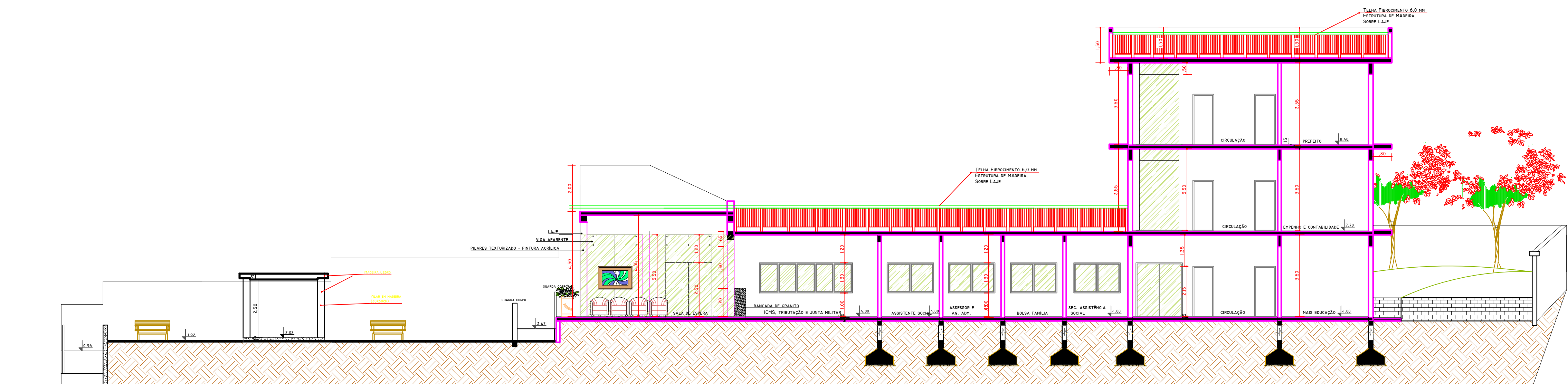
CORTE TRANSVERSAL BB'
