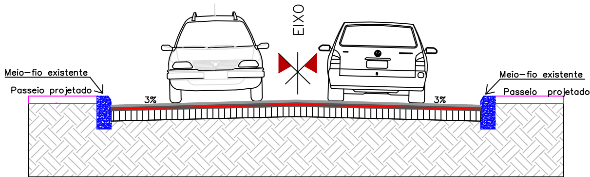
SEÇÃO TIPO ERNESTO SEBASTIANI SEM ESCALA
