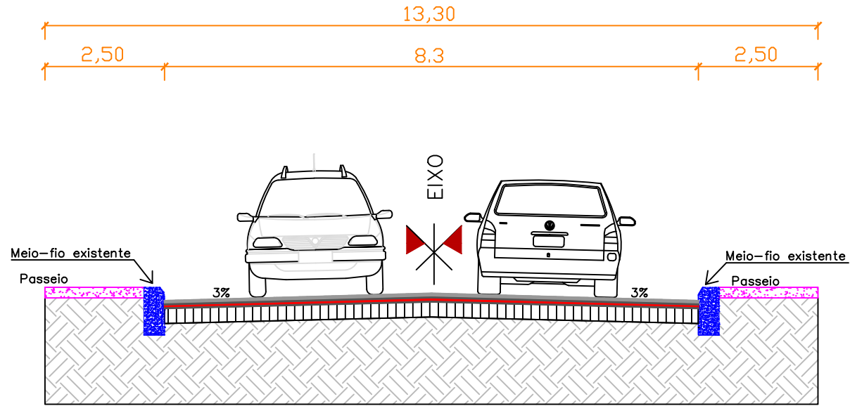
SEÇÃO DE PAVIMENTAÇÃO NA RUA ALOÍSIO SCHERER CORTE A-A SEM ESCALA
