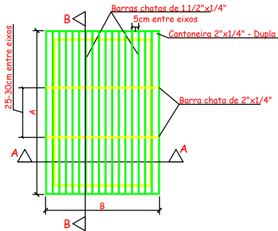
PLANTA - GRELHA
