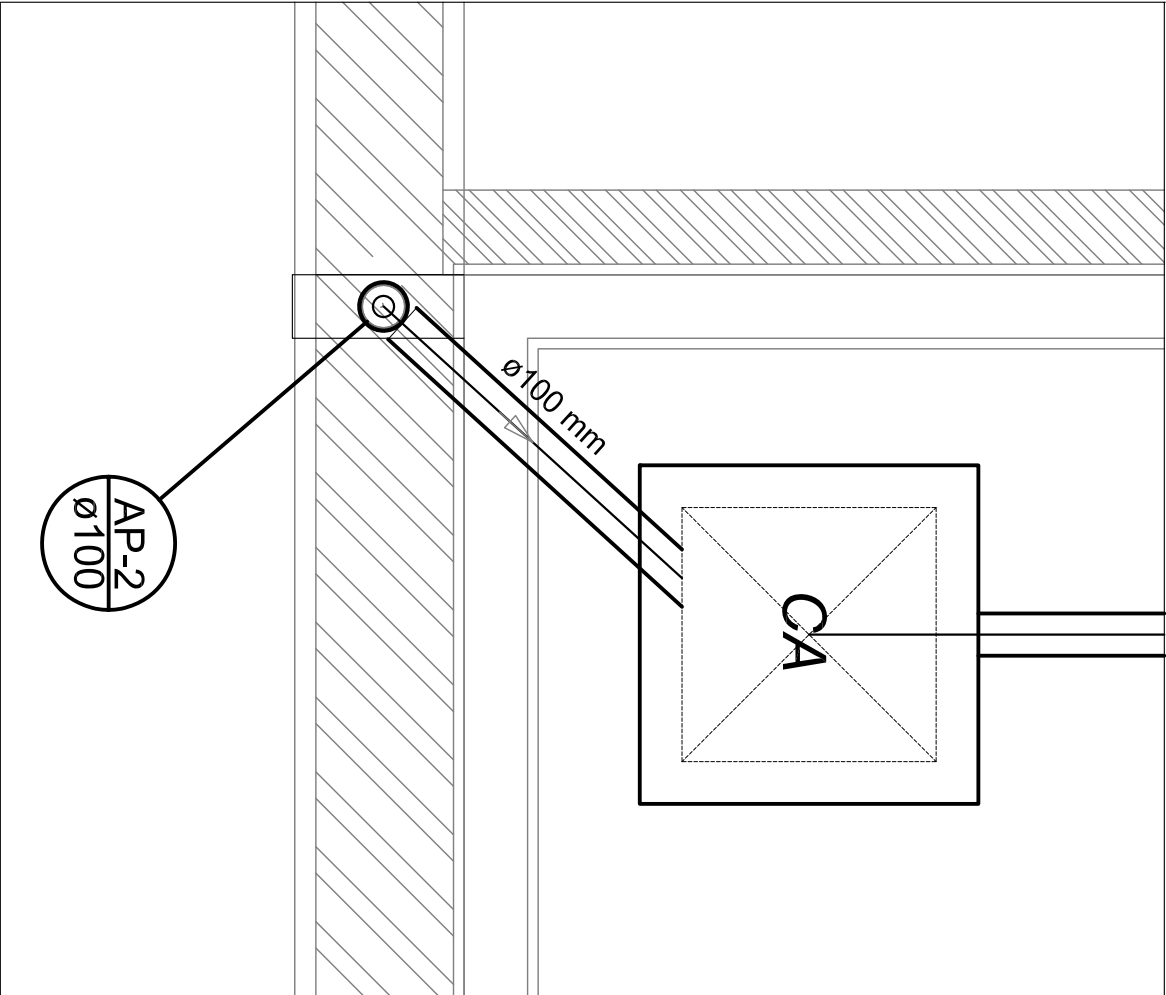
Detalhe S1 escala 1:20
