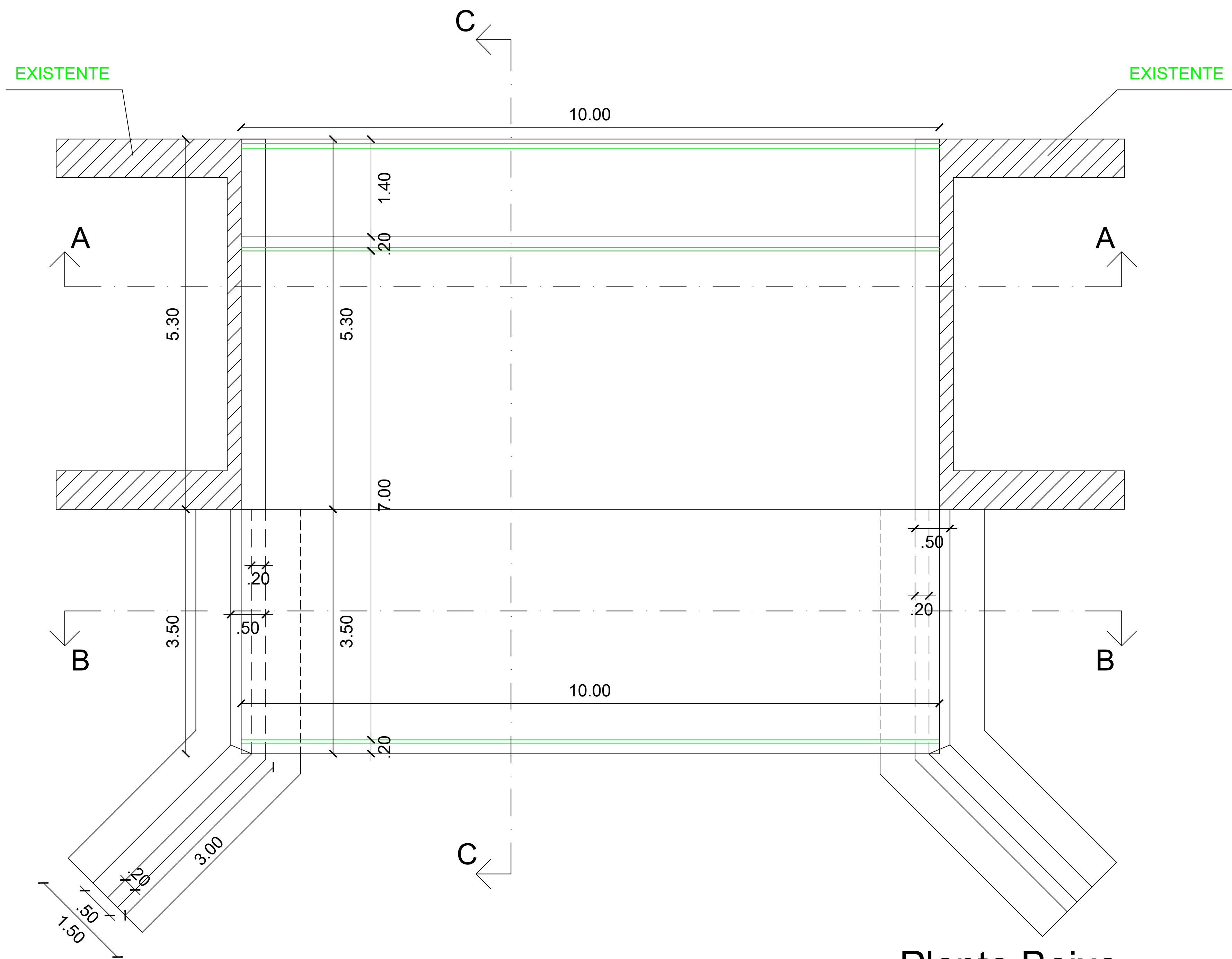
Planta Baixa
