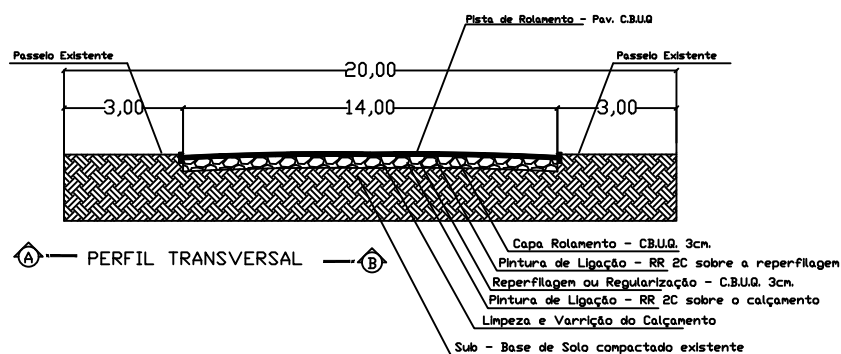
PERFIL TRANSVERSAL PAVIMENTAÇÃO C.B.U.Q (CAPEAMENTO)- SOBRE PAVIMENTO DE CALÇAMENTO
