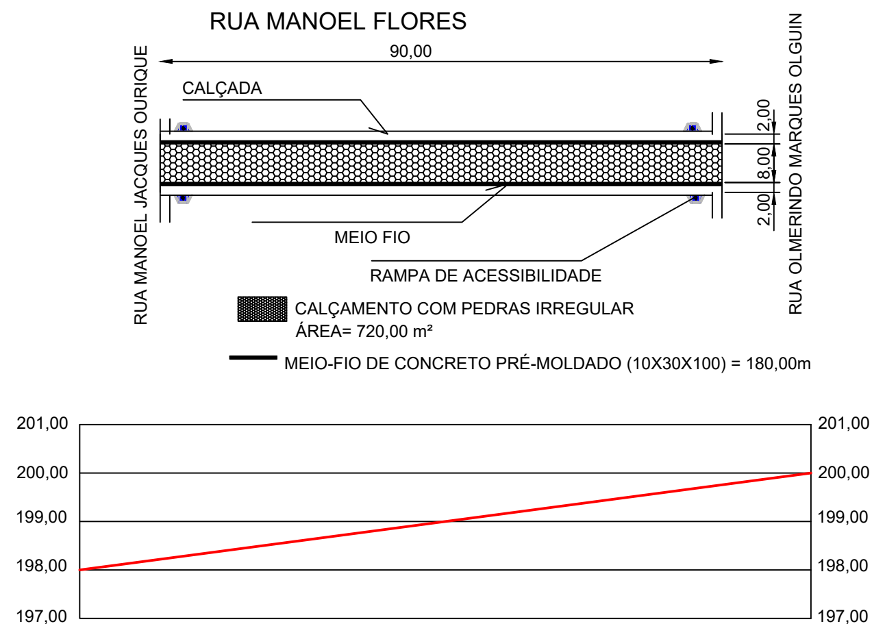
PERFIL LONGITUDINAL DA VIA
