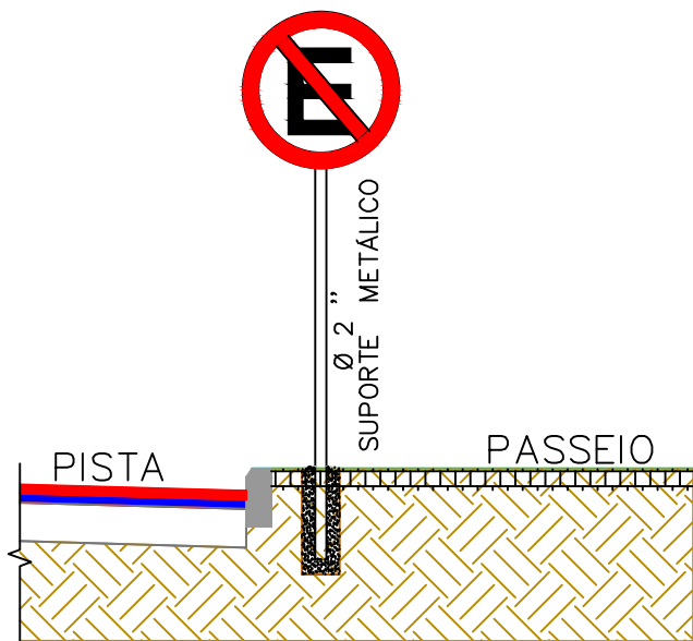
DETALHE INST. PLACAS SEM ESCALA R-6a PROIBIDO ESTACIONAR (L=0,50m)
