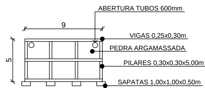
VISTA FRONTAL (LESTE)
