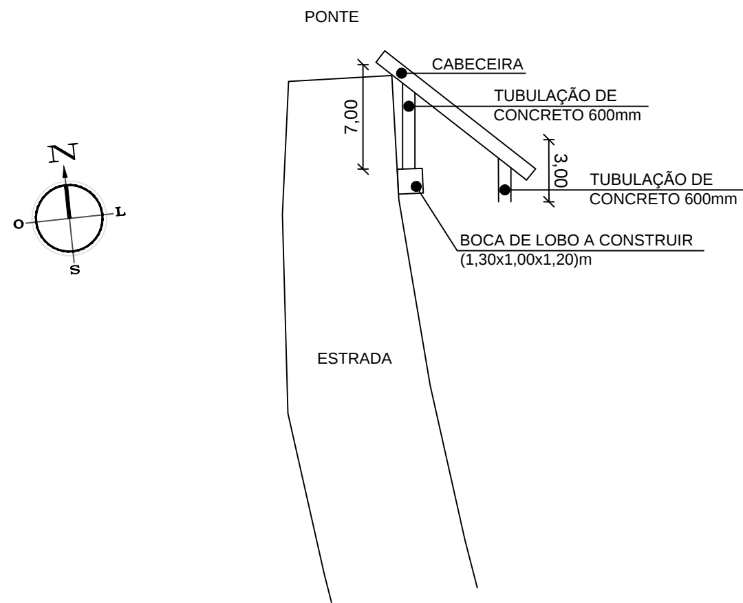
VISTA SUPERIOR
