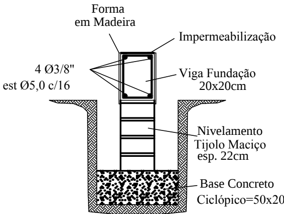
DETALHE FUNDAÇÃO Esc.:1/20
