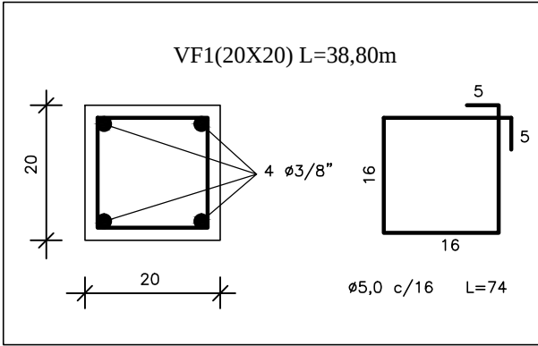
DETALHE ARMADURA VIGAS DE FUNDAÇÃO Esc.: 1/10
