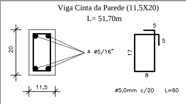
DETALHE ARMADURA VIGAS SUPERIORES Esc.: 1/10
