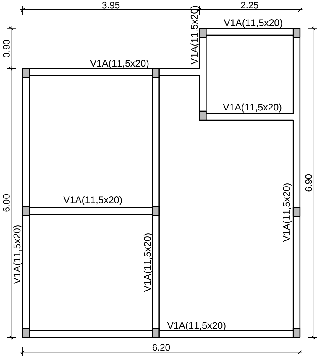
PROJETO ESTRUTURAL VIGAS SUPERIORES (CINTA DA PAREDE) ESC.:1/50
