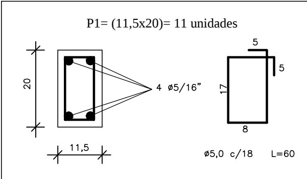
DETALHE ARMADURA PILARES Esc.: 1/10
