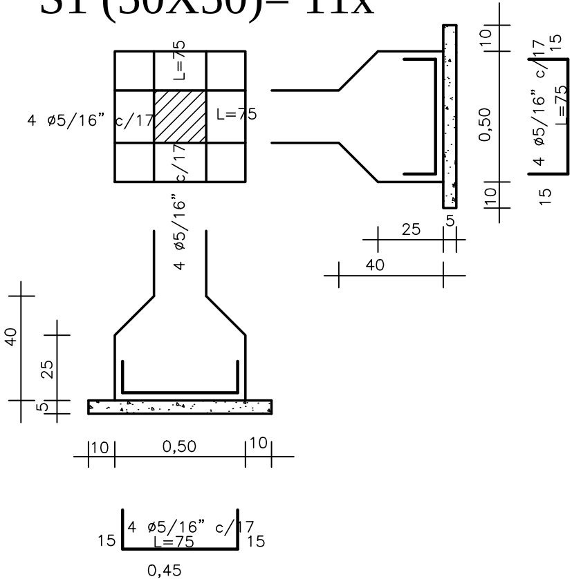
DETALHE ARMADURA SAPATA Esc.:1/25
