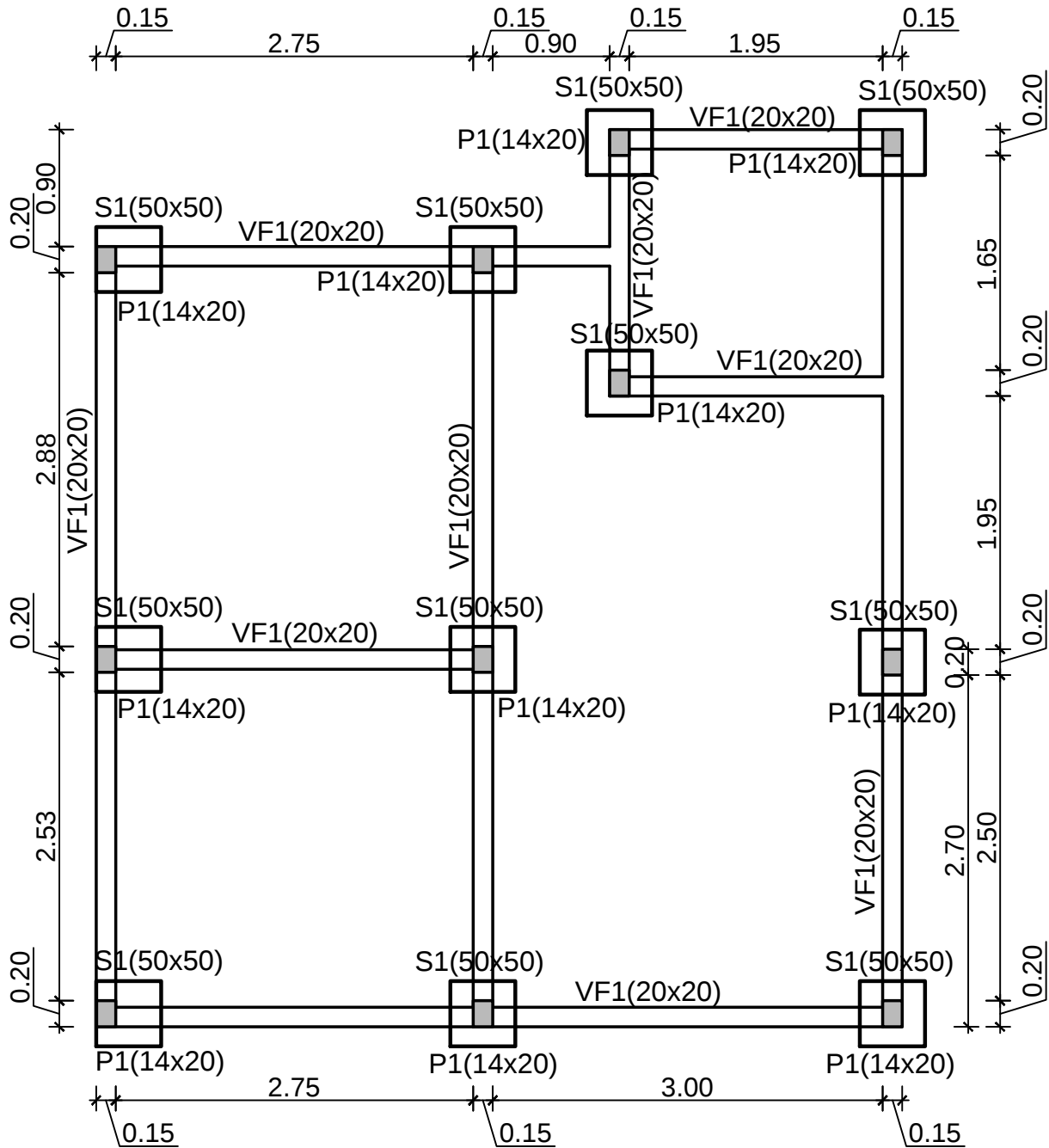
PROJETO ESTRUTURAL LOCAÇÃO SAPATAS, PILARES E VIGAS DE FUNDAÇÃO ESC.: 1/50
