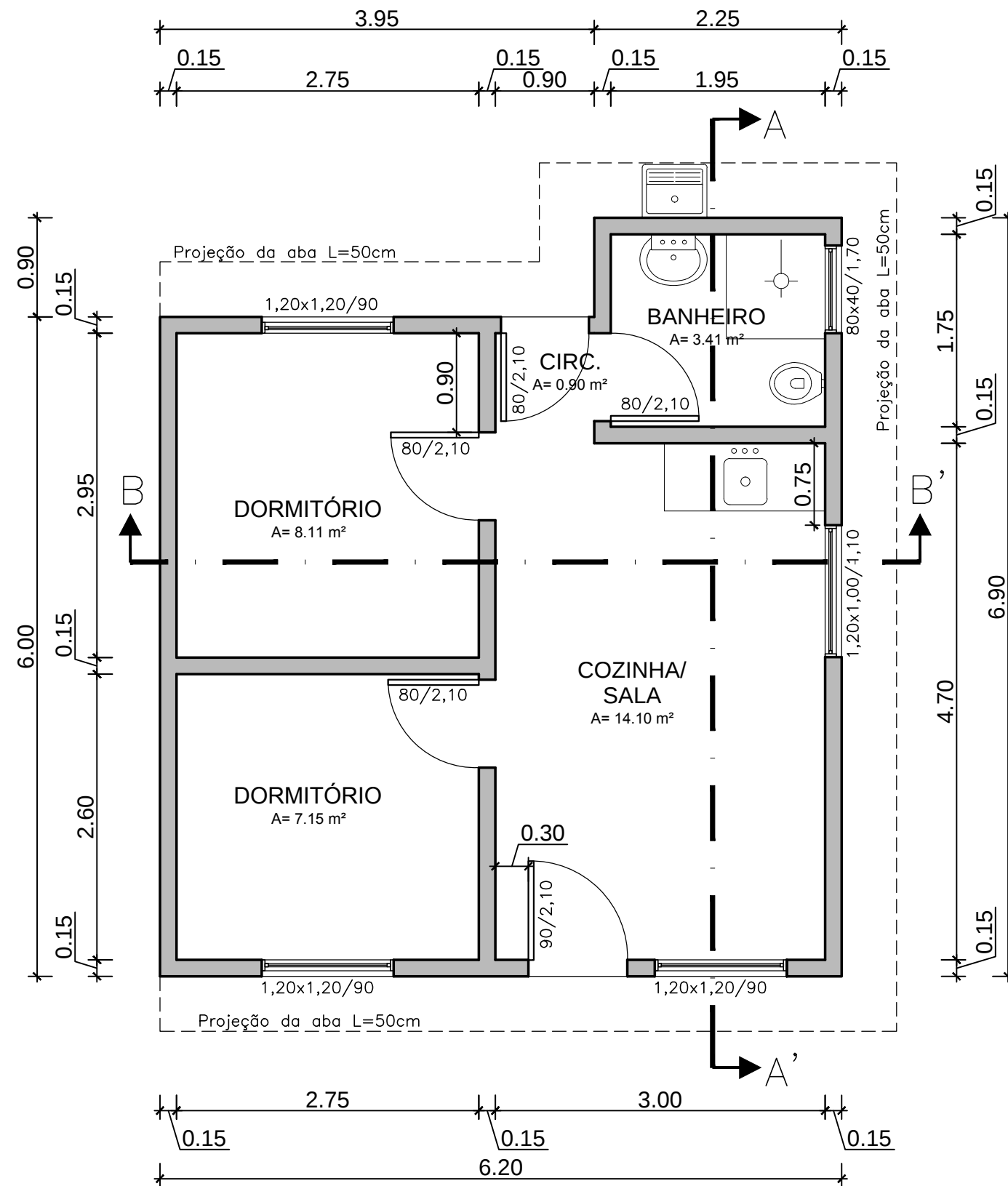
PLANTA BAIXA ÁREA TOTAL= 39.22 m² Esc.: 1/50
