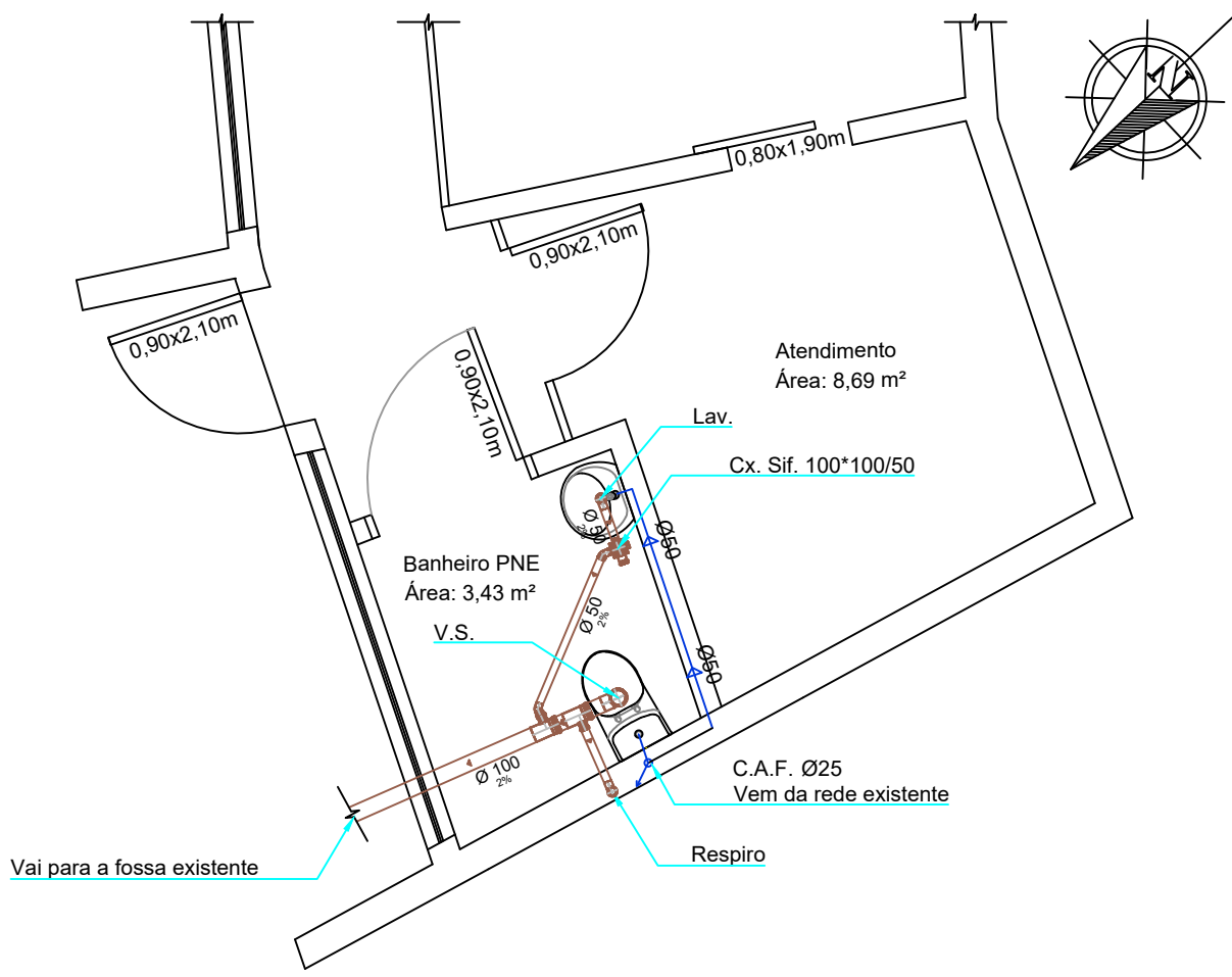
Instalações Hidrossanitárias - Banheiro PNE Pavimento Inferior Escala 1:50
